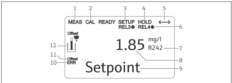
15 LC zaslon odašiljača
