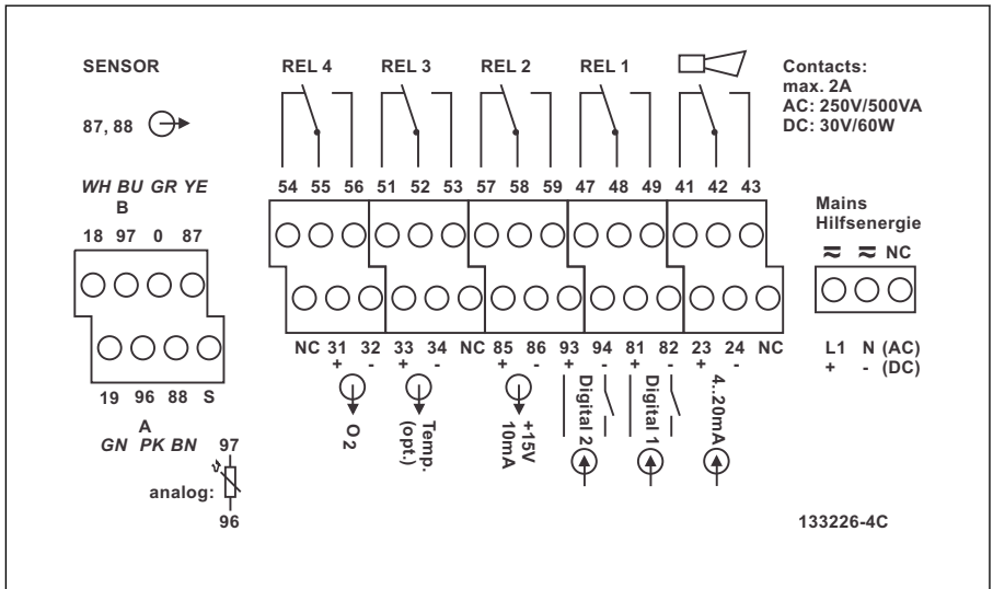
11 Liquisys M naljepnica pretinca priključka, verzija WX/WS
