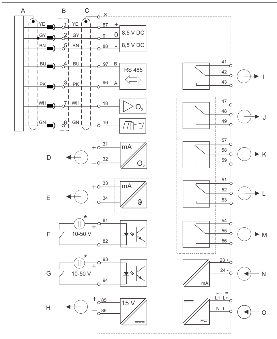
10 Električni priključak Liquisys M COM223/253 u verziji WX ili WS
