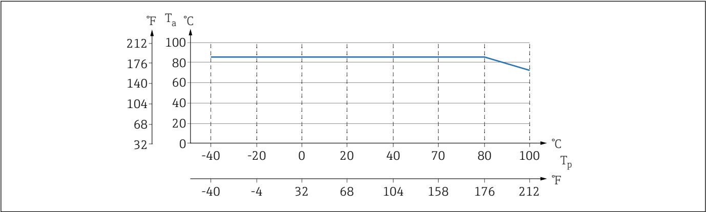
12 Les valeurs sont valables pour un montage vertical sans isolation.
