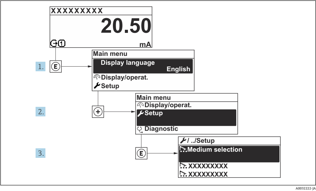
図 16 「設定」メニューへのナビゲーション（現場表示器の表示例）
