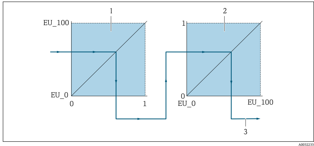
図 18 アナログ入力ブロックの測定値のスケーリング
