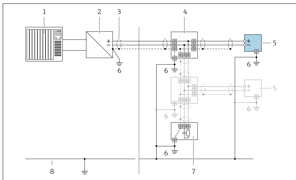
図 8 FOUNDATION Fieldbus の接続例
