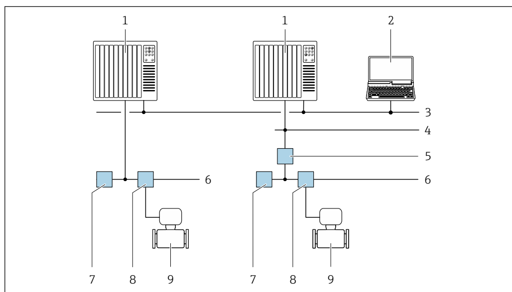
図 14 FOUNDATION Fieldbus ネットワークを介したリモート操作のオプション
