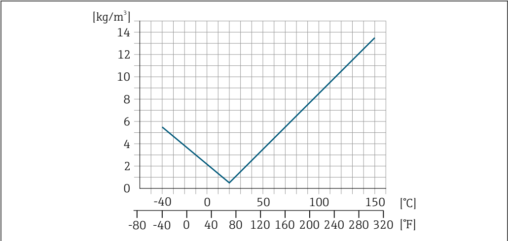
図 25 現場密度調整、例：+20 °C (+68 °F) 時
