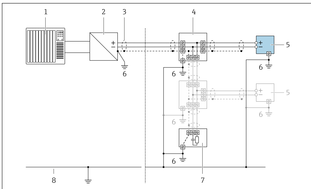
図 11 FOUNDATION Fieldbus の接続例
