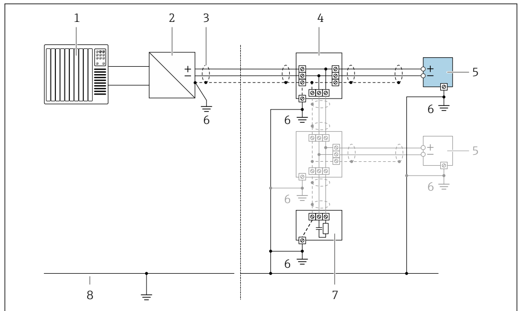
20 Exemplo de conexão para o FOUNDATION Fieldbus
