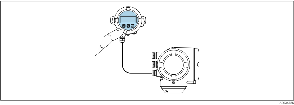
39 Operação através do display remoto e do módulo de operação DKX001
