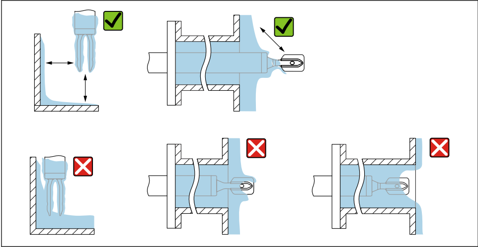
☞ 7 고점성 프로세스 유체용 설치 예
