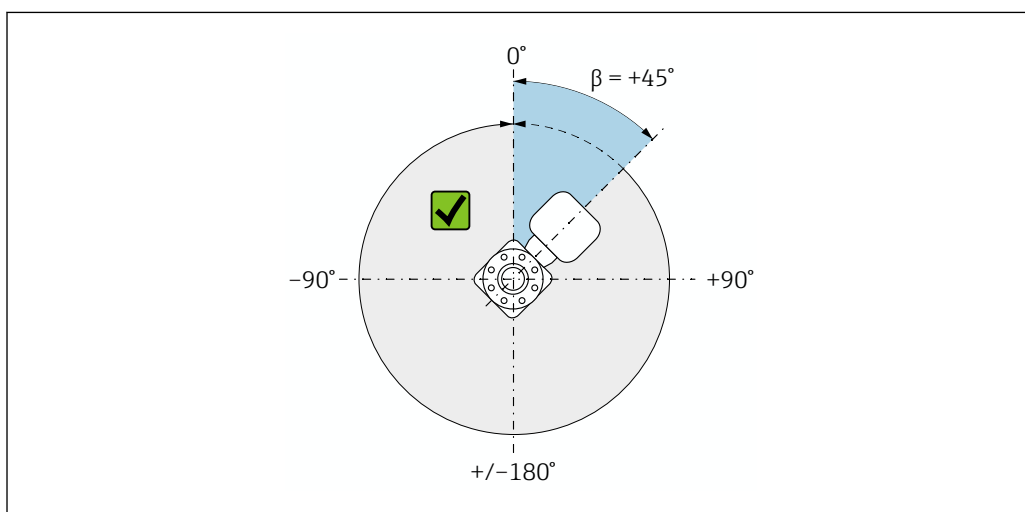
8 Вид сверху, по направлению потока
