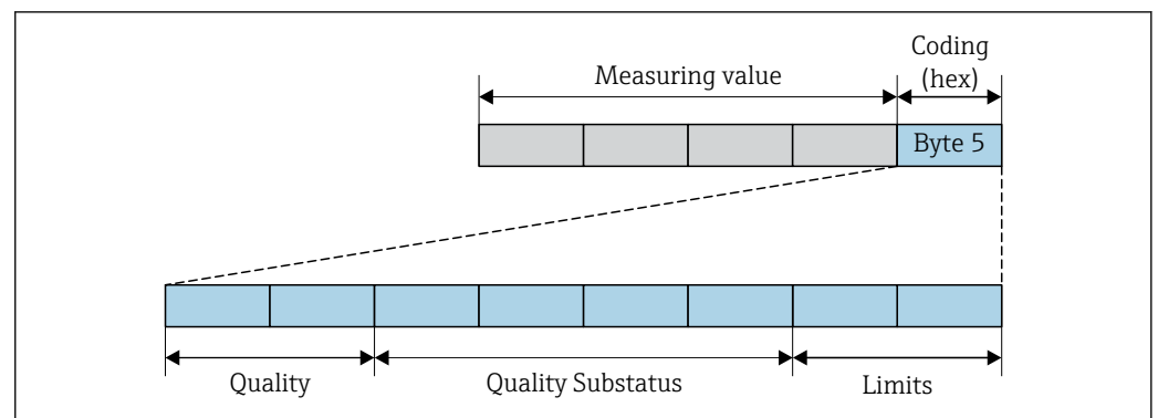
32 Структура байта кодирования
