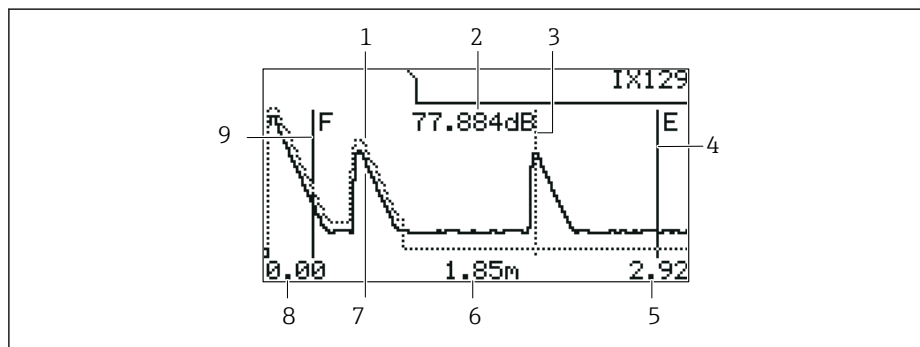
64 Огибающая кривая на локальном дисплее
