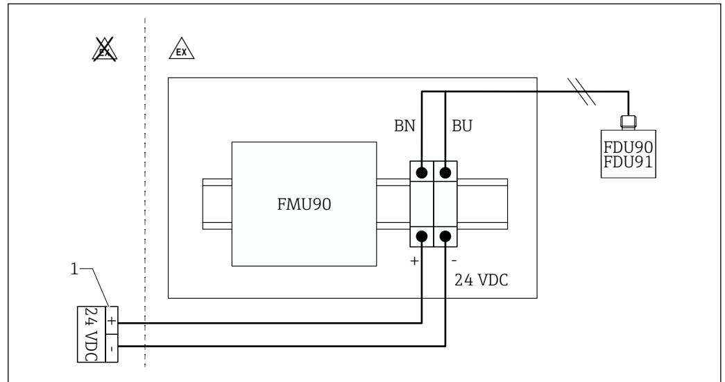
31 Подключение подогревателя датчика к прибору в алюминиевом полевым корпусе
