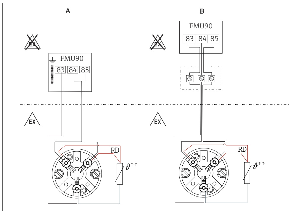
38 Подключение датчика Omnigrad S TR61 во взрывоопасной зоне
