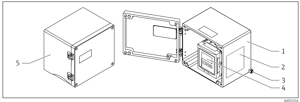
2 Компоненты прибора Prosonic S в алюминиевом полеовом корпусе
