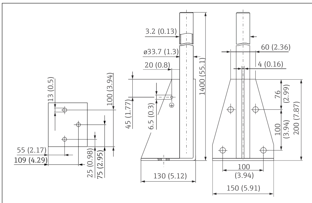
68 Размеры. Единица измерения мм (дюйм)
