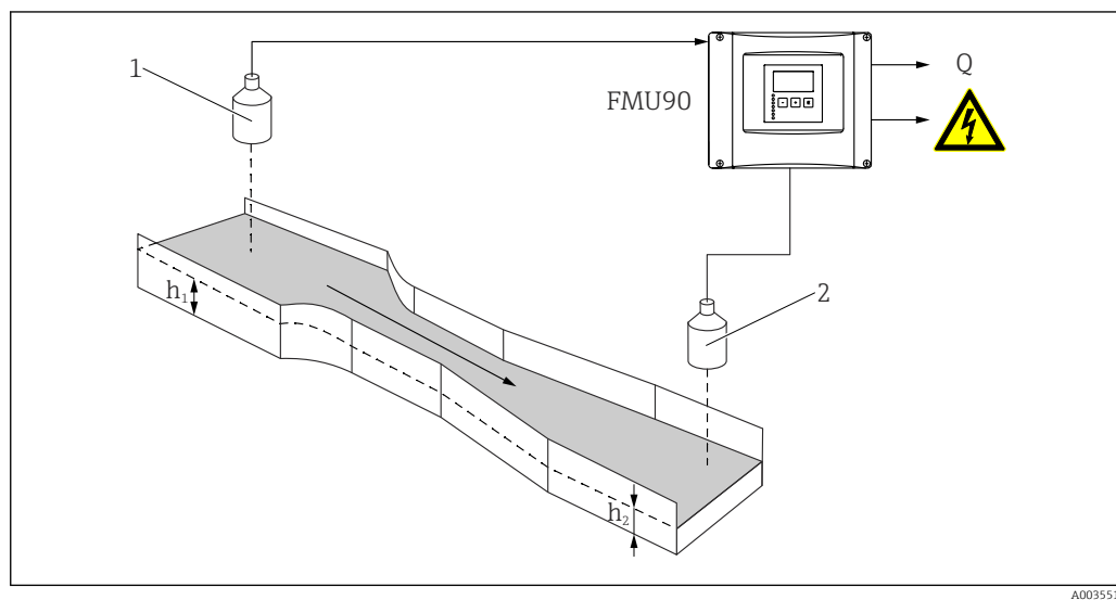
49 Обнаружение обратного потока с помощью двух ультразвуковых датчиков
