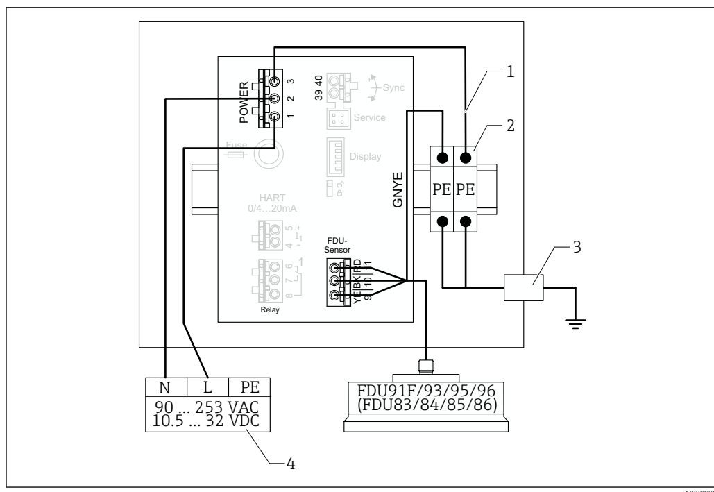
27 Выравнивание потенциалов металлических датчиков для прибора в алюминиевом полевым корпусе
