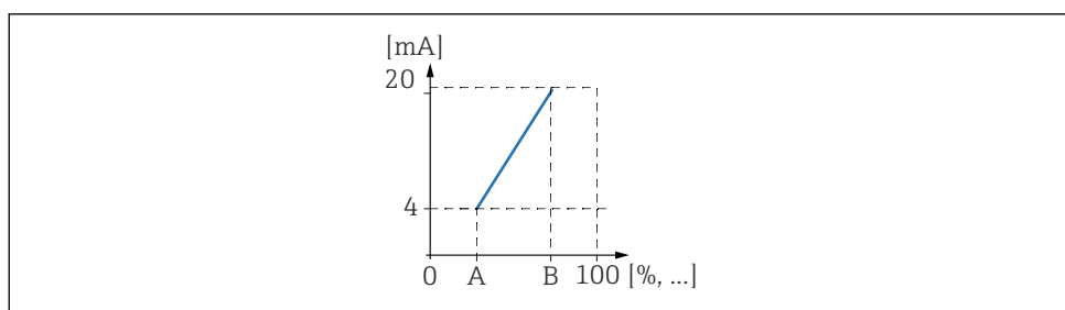
62 Принцип работы функции перестройки силы тока
