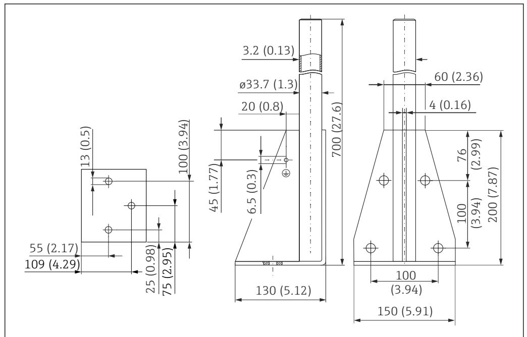
67 Размеры. Единица измерения мм (дюйм)
