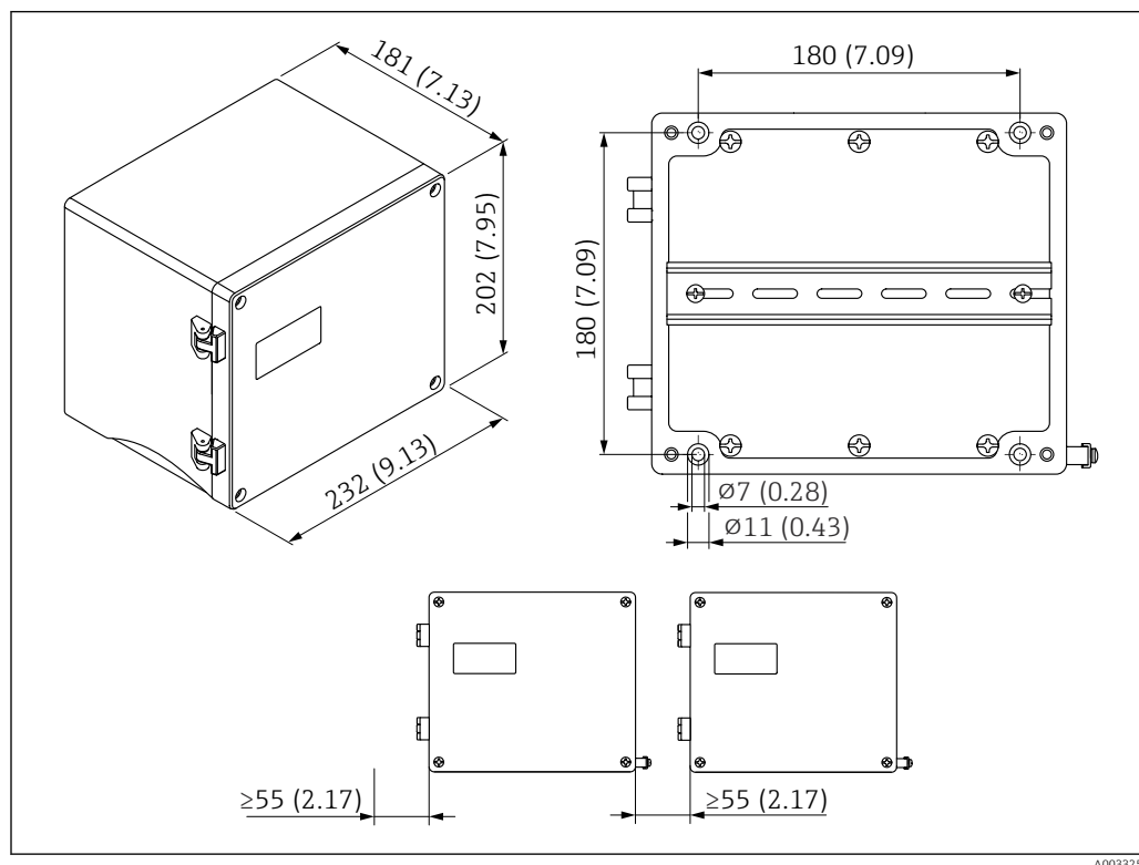
9 Размеры прибора Prosonic S в алюминиевом полевым корпусе. Единица измерения мм (дюйм)
