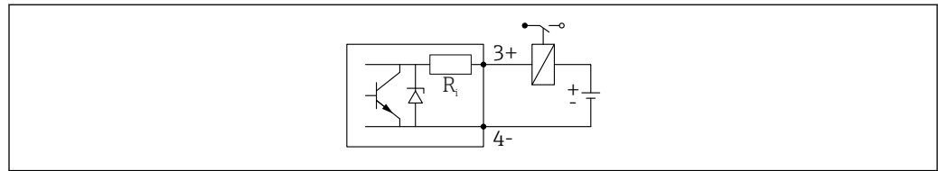
19 Anschluss eines Relais
