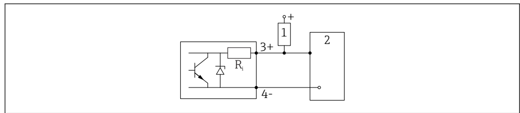
20 Anschluss an einen Digitaleingang
