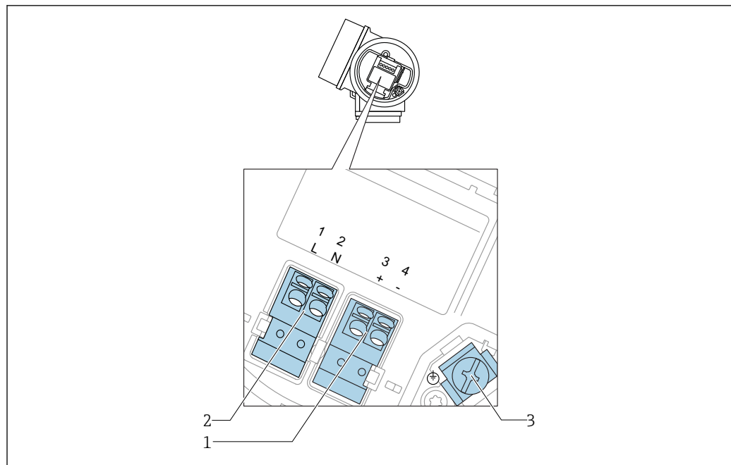
17 Klemmenbelegung 4-Draht: 4-20 mA HART (90 ... 253 V AC )
