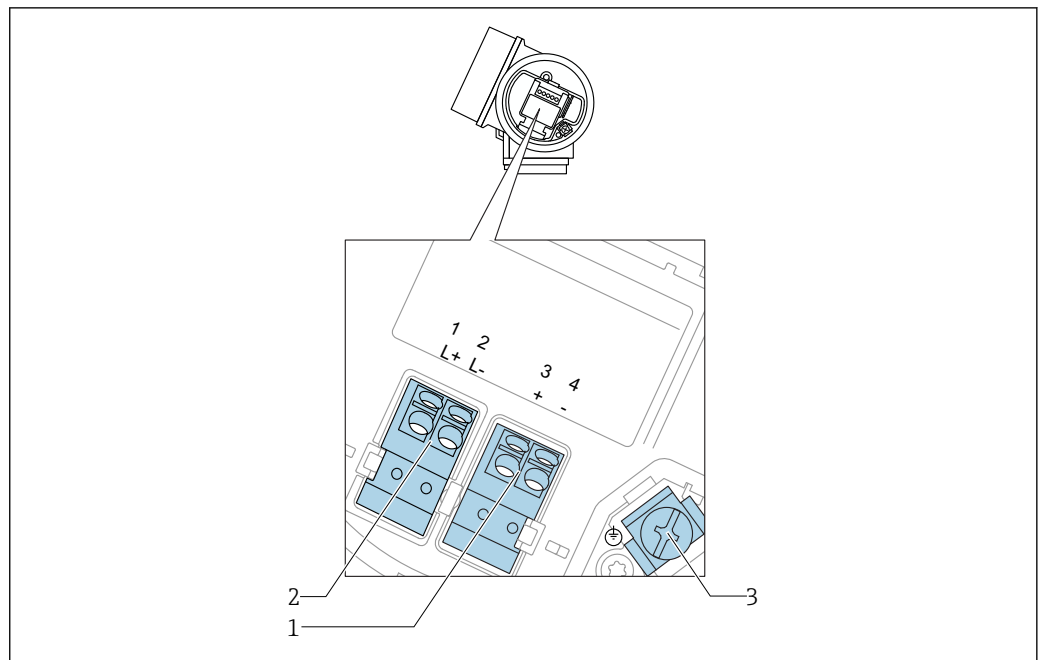
15 Klemmenbelegung 4-Draht: 4-20 mA HART (10,4 ... 48 V DC )
