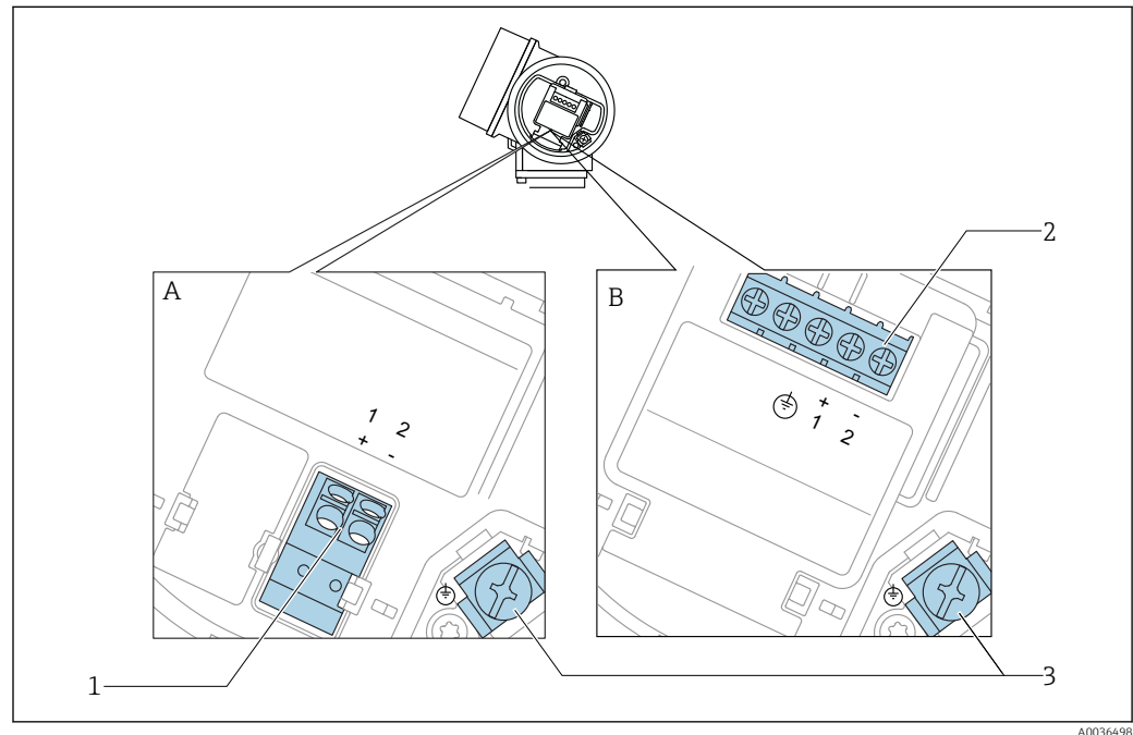
9 Klemmenbelegung 2-Draht: 4-20 mA HART
