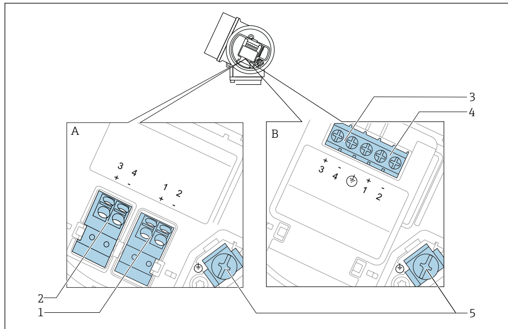
13 Klemmenbelegung 2-Draht: 4-20 mA HART, 4-20 mA
