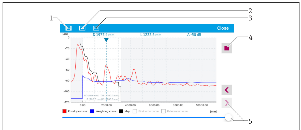
33 Hüllkurvendarstellung (Beispiel) in SmartBlue bei iOS
