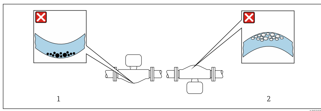
☒ 14 Position du capteur avec tube de mesure coudé
