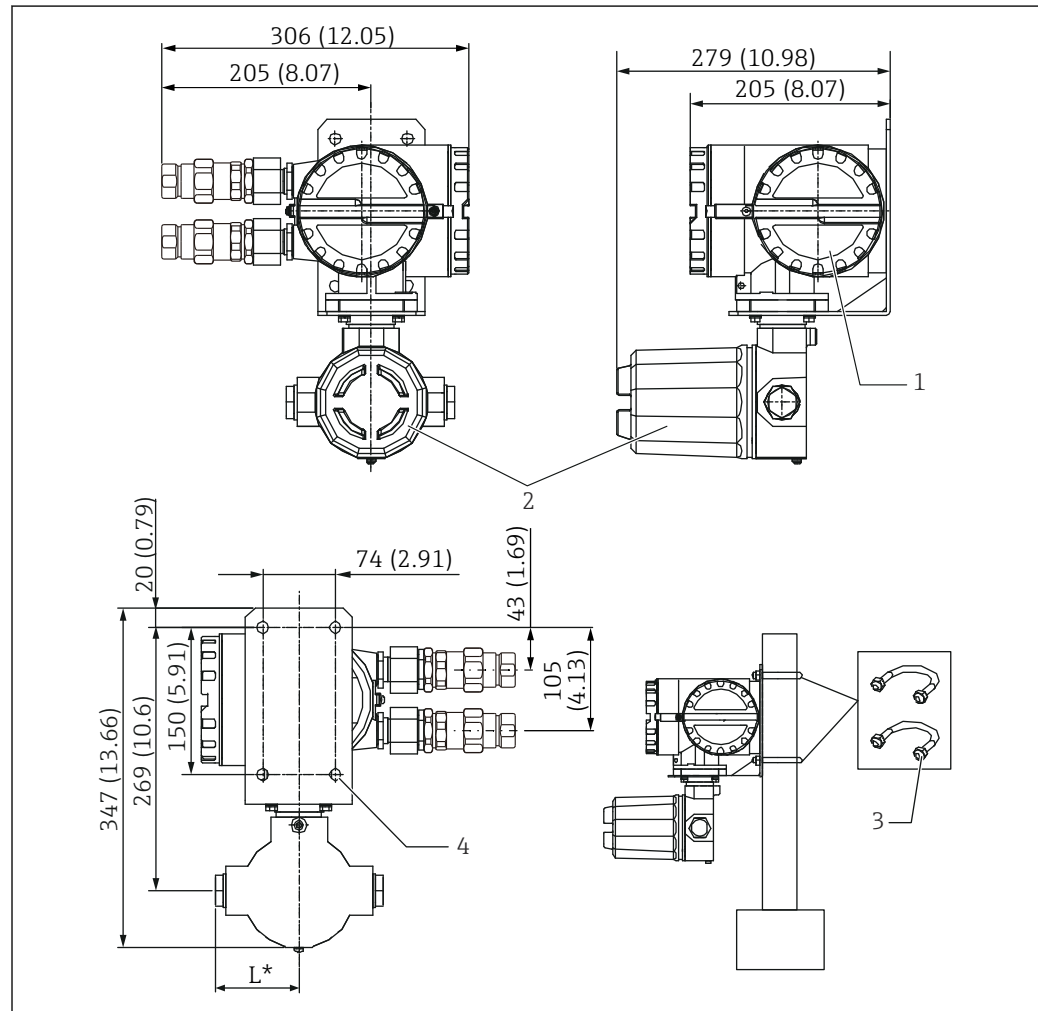
图 10 NRR261 的外形尺寸示意图。测量单位 mm (in)
