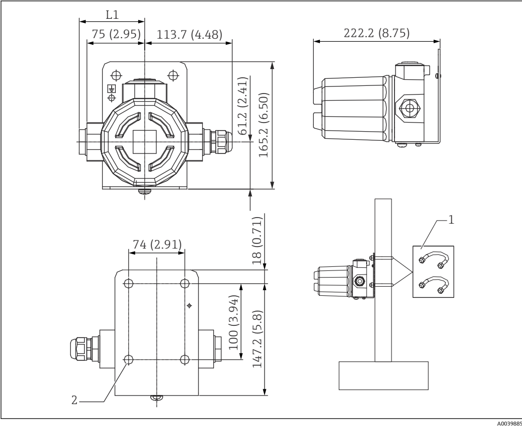
图 12 本安防爆型 (Ex [ia]) 传感器数据转换盒的外形尺寸示意图。测量单位 mm (in)
