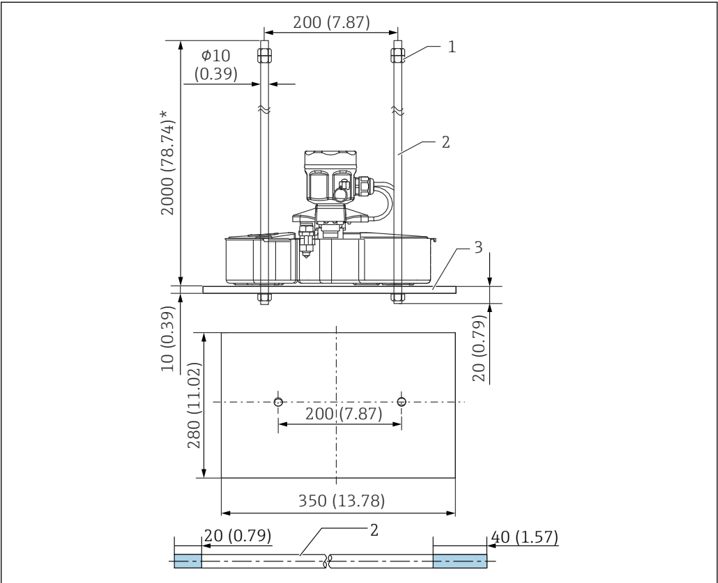
图 15 浮子导杆
