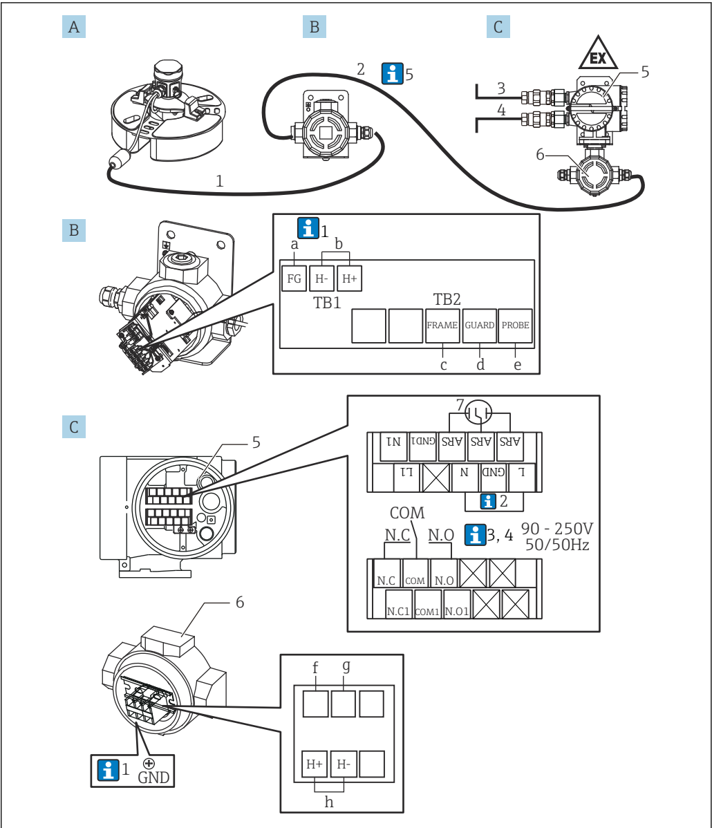
图 6 本安隔爆型 (Ex d [ia]) 转换器 NRR261-5 接线示意图
