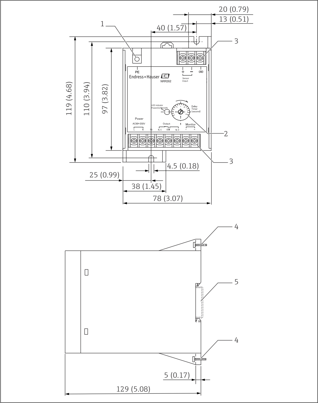
图 11 NRR262 的外形尺寸示意图。测量单位 mm (in)
