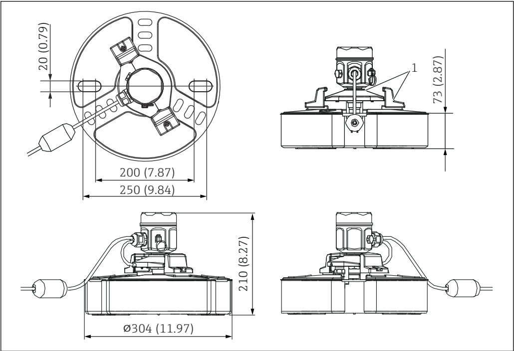
图 9 NAR300 浮子开关的外形尺寸示意图
