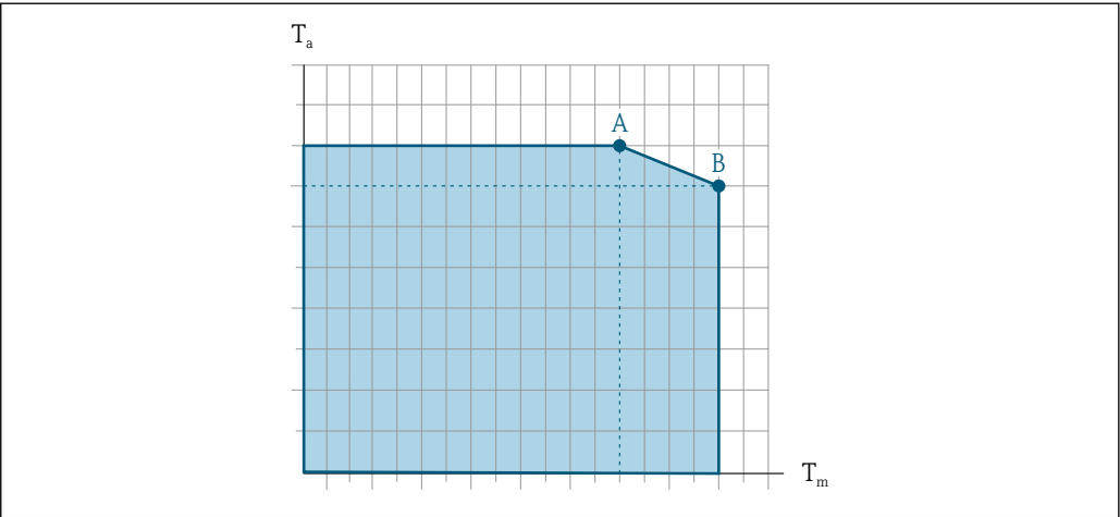
33 Rappresentazione esemplificativa, valori nella tabella sottostante. T_a Temperatura ambiente T_m Temperatura del fluido A Temperatura del fluido massima consentita T_m con T_{a\,max} = 60\,^{\circ}\text{C} (140 °F); temperature del fluido superiori T_m richiedono una temperatura ambiente ridotta T_a B Temperatura ambiente massima consentita T_a per la temperatura del fluido massima specificata T_m del sensore
