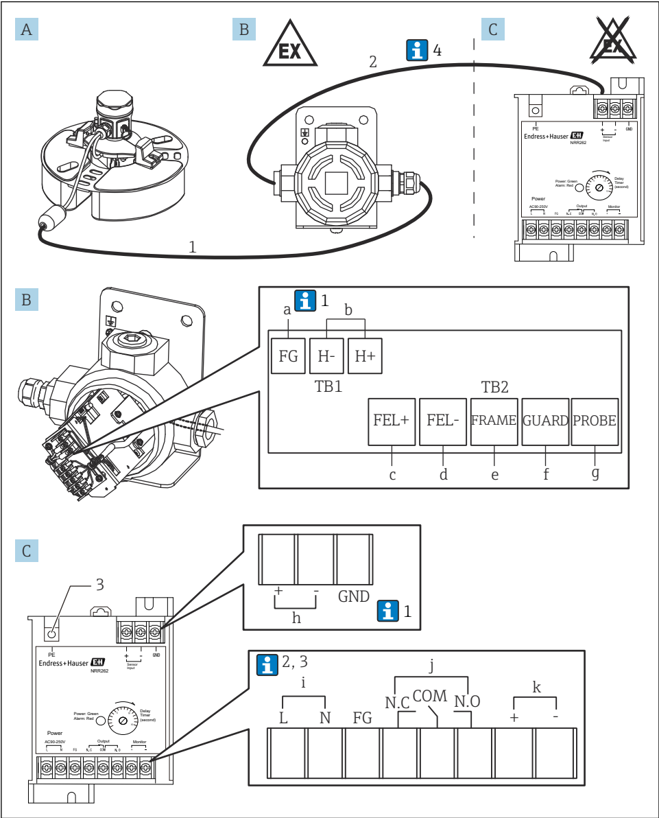
15 本安防爆型 (Ex iaI) 转换器 NRR262-4/A/B/C 接线示意图
