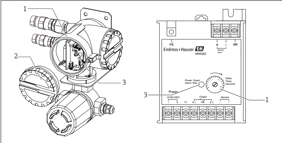
图 13 报警输出继电器
