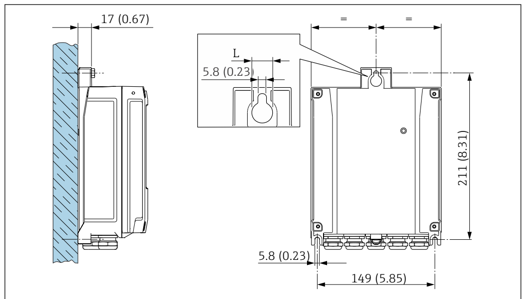
12 工学単位 mm (in)
