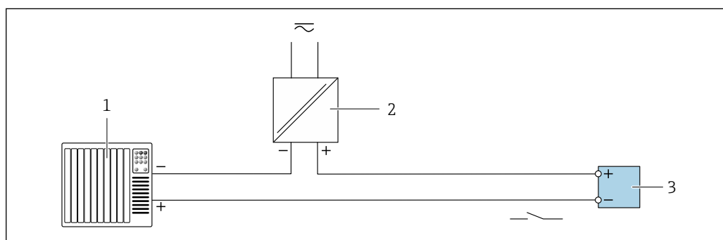
図 24 スイッチ出力（パッシブ）の接続例
