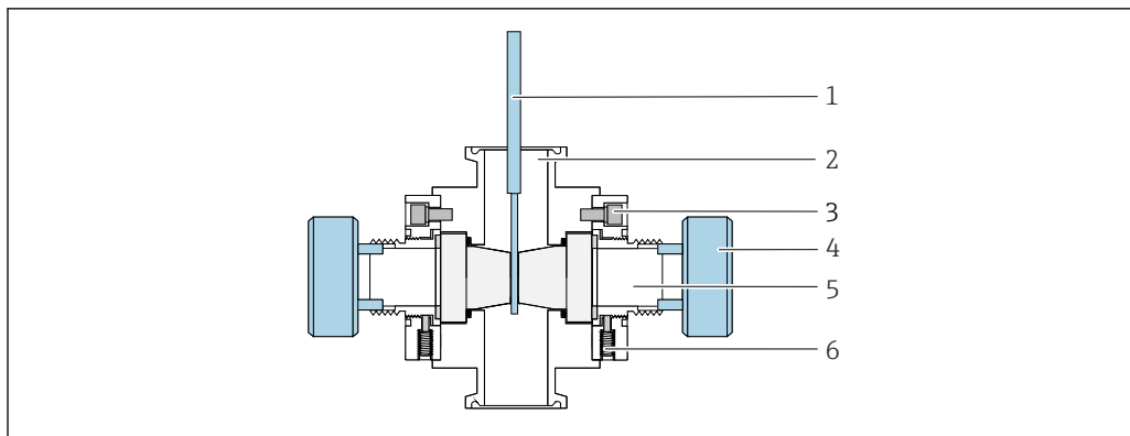
5 Sklop s POPL funkcijom, presjek
