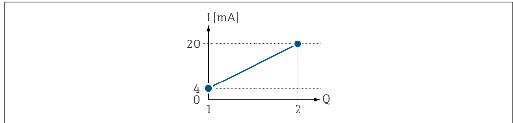
図 2 測定範囲
