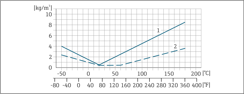
1 Ajustage sur site de la masse volumique, par exemple à +20 °C (+68 °F) 2 Étalonnage de la masse volumique étendue
