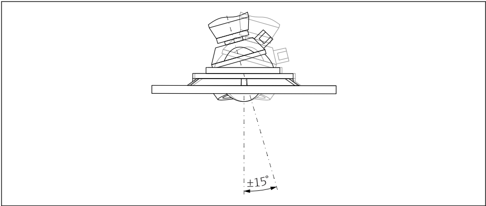
図 2 角度調節器付きフラッシュマウントアンテナ
