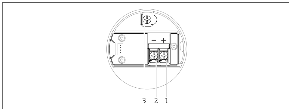
図 15 端子部の端子の割当て ; 4~20 mA HART ; デュアルコンパートメントハウジング L 字型
