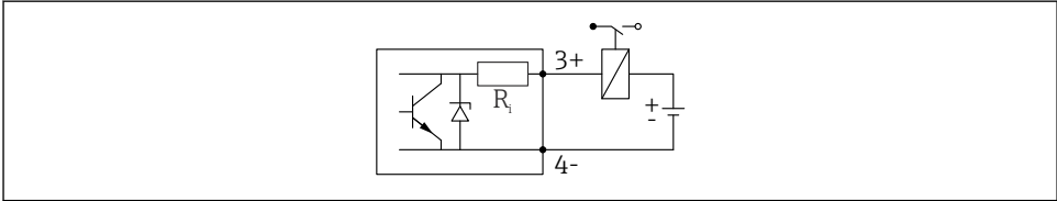
図 8 リレーの接続例
