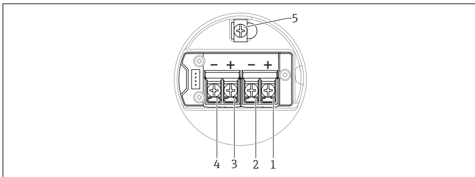
図 17 端子部の端子の割当て ; 4~20 mA HART、スイッチ出力 ; デュアルコンパートメントハウジング L 字型
