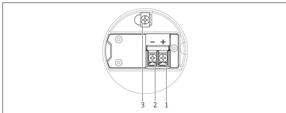
図 12 端子部の端子の割当て；4～20 mA HART；デュアルコンパートメントハウジング
