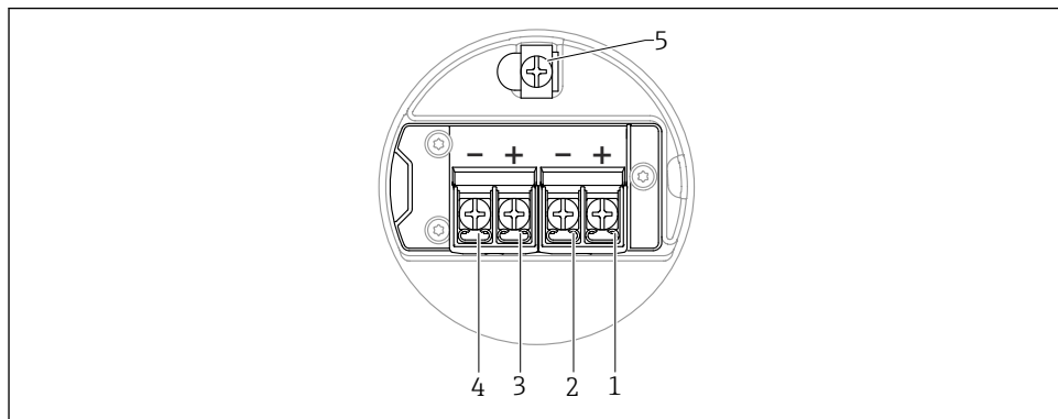
図 13 端子部の端子の割当て ; 4~20 mA HART + 4~20 mA アナログ ; デュアルコンパートメントハウジング
