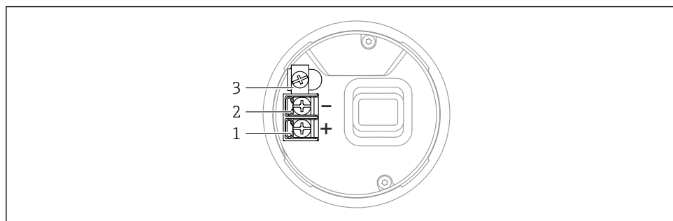
図 11 端子部の接続端子と接地端子（シングルコンパートメントハウジング）
