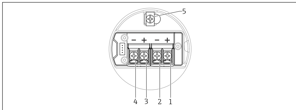
図 16 端子部の端子の割当て ; 4~20 mA HART + 4~20 mA アナログ ; デュアルコンパートメントハウジング L 字型
