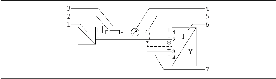
図 7 4～20 mA HART、スイッチ出力の機能図
