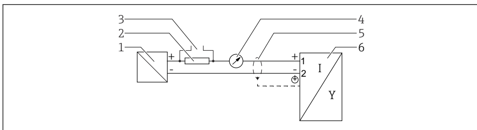
図 6 機能図 4～20 mA HART
