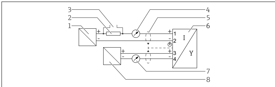
図 10 4~20 mA HART + 4~20 mA アナログの機能図
