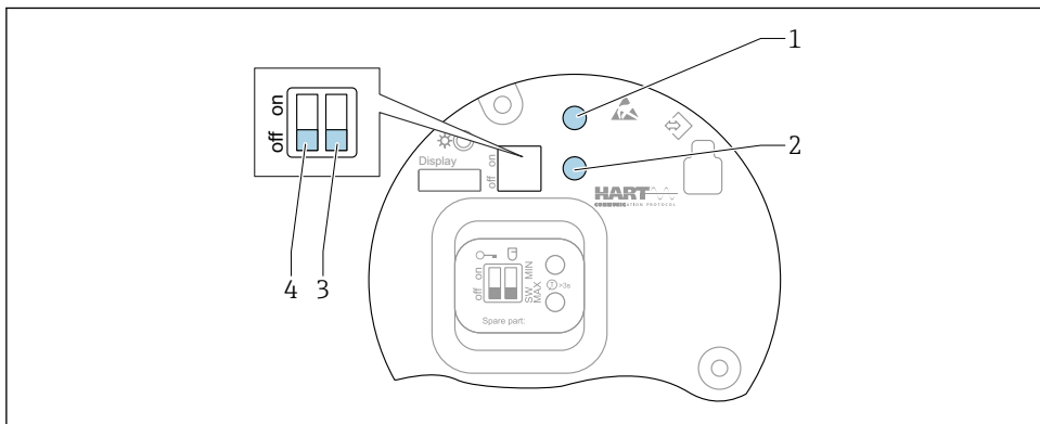
図 18 HART エレクトロニックインサート上の操作キーおよび DIP スイッチ
