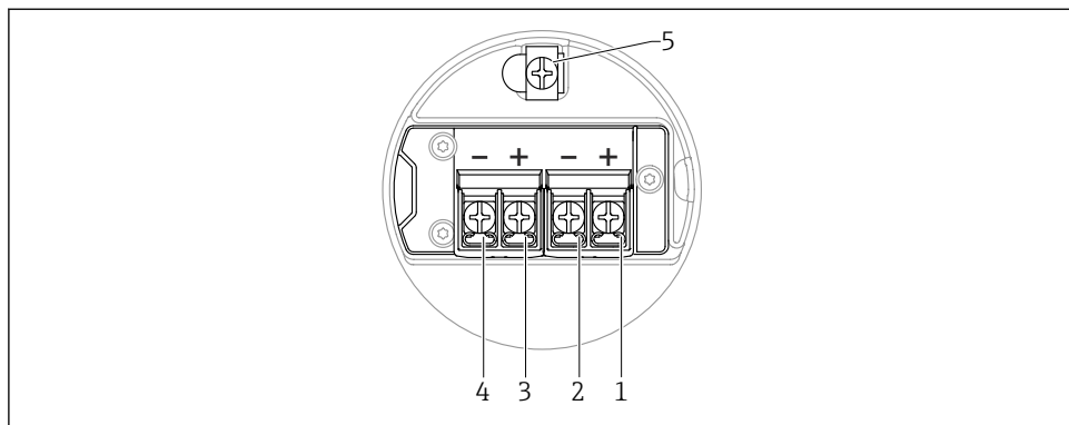
図 14 端子部の端子の割当て ; 4~20 mA HART、スイッチ出力 ; デュアルコンパートメントハウジング
