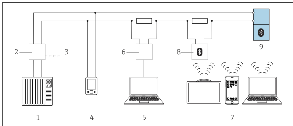
図 21 HART プロトコル経由のリモート操作用オプション
