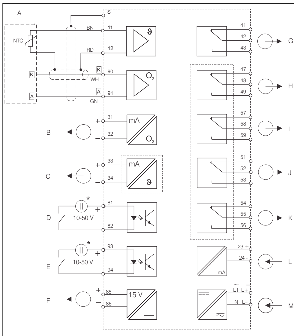
3 Elektrischer Anschluss des Messumformers in Ausführung DX oder DS
