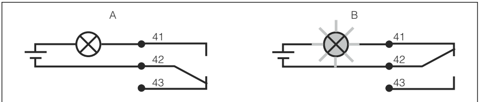
10 Empfohlene Fail-Safe-Schaltung für den Alarmkontakt
