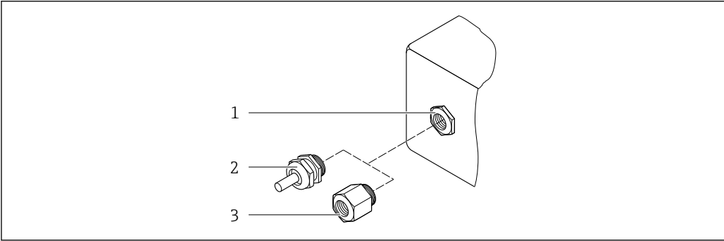
41 Entradas de cable/prensaestopas posibles 1 Rosca interna M20 × 1,5 2 Prensaestopas M20 × 1,5 3 Adaptador para entrada de cable con rosca interna G ½" o NPT ½"
