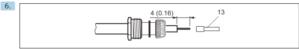
9 Terminering af pH-tilslutningskablet i BNC-vinkelstikproppen. Dimensioner i mm (inch)
