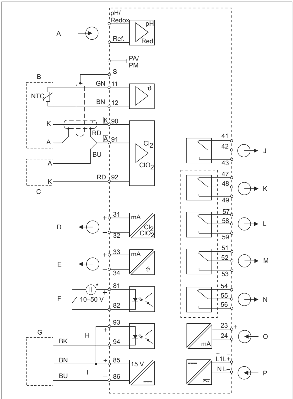
3 Elektrisk tilslutning af transmitteren (version 1)
