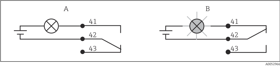
12 Anbefalet fejlsikker afbryder for alarmkontakten
