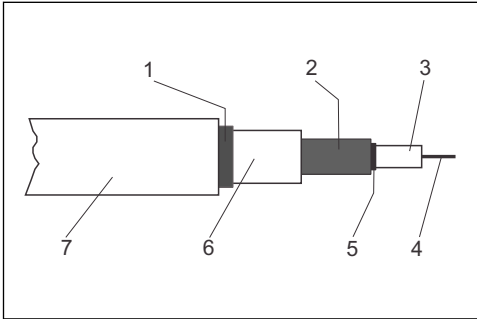
11 Kabelstruktur CYK71
