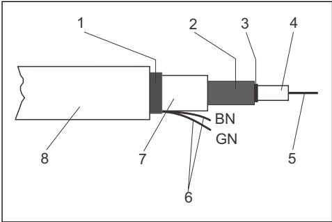
10 Kabelstruktur CMK
