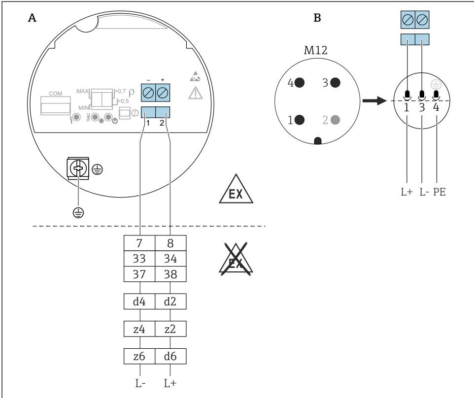
图 24 电子插件 FEL67: PFM 输出
