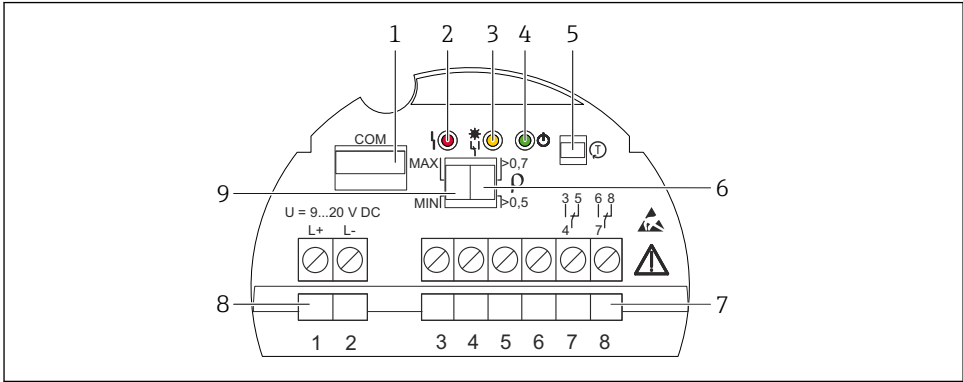
图 29 实例：电子插件 FEL64DC
