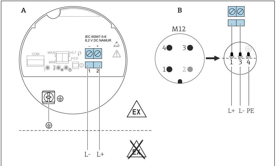
26 电子插件 FEL68: 两线制连接, NAMUR 信号 ( \geq 2.2 \text{ mA} / \leq 1.0 \text{ mA} )
