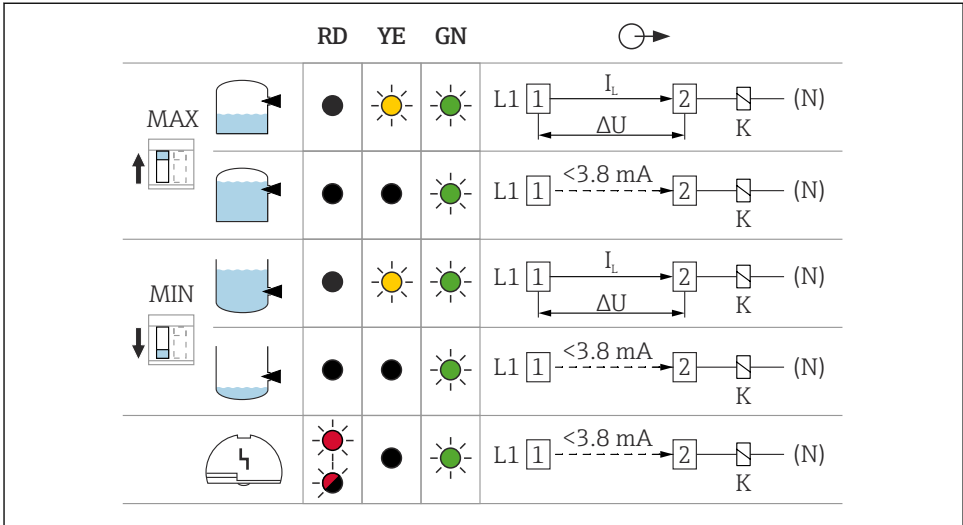
图 16 电子插件 FEL61 的继电器响应和故障信号
