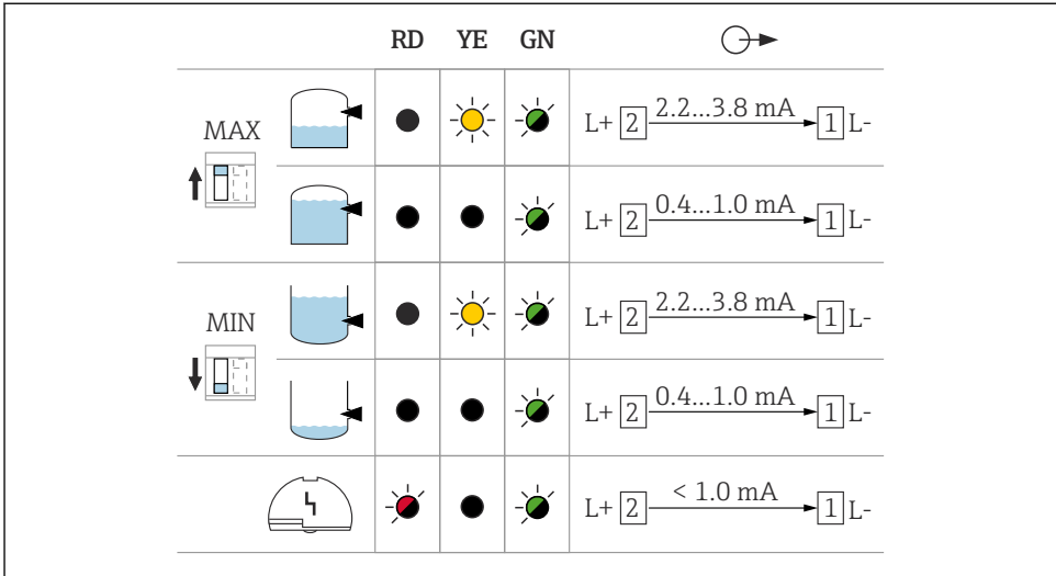
图 27 电子插件 FEL68 的开关量输出和信号传输
