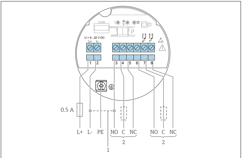
图 22 电子插件 FEL64 DC: 直流连接型, 带继电器输出
