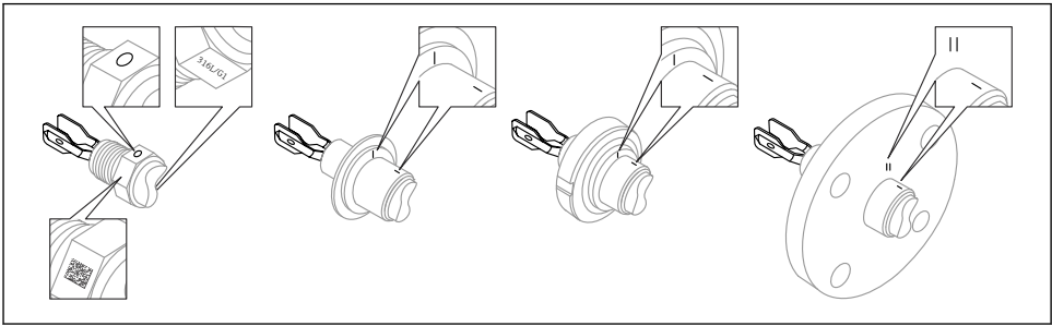
图 9 参照标记水平安装在罐体中时的音叉位置
