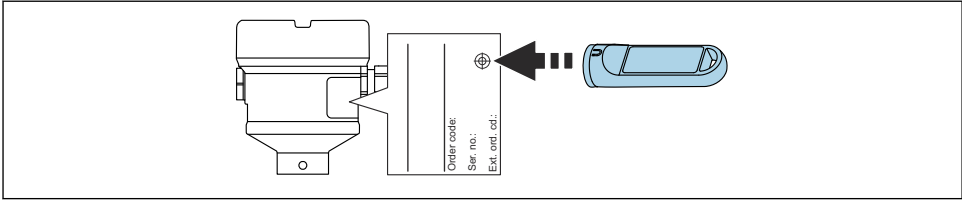
图 32 使用测试磁铁进行功能测试
