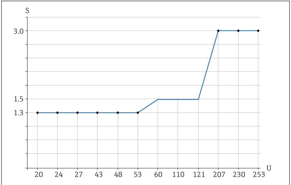
图 17 负载的推荐最小持续功率/额定功率
