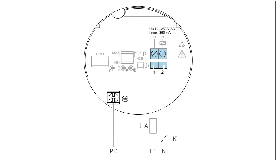
15 FEL61 电子插件：两线制连接，交流 AC 型
