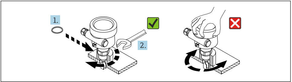
图 11 旋转拧入设备
