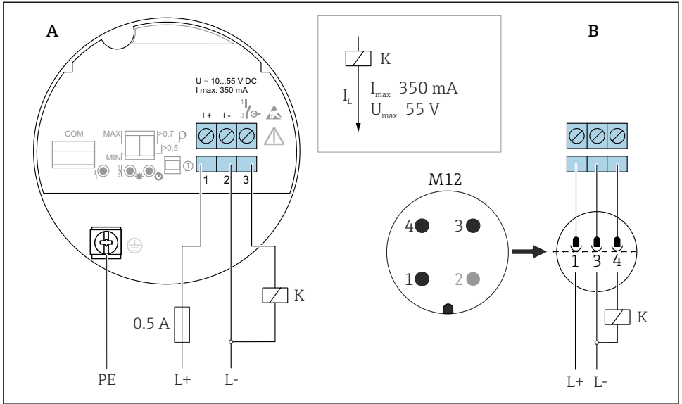
图 18 电子插件 FEL62: 三线制连接, 直流 DC-PNP 型
