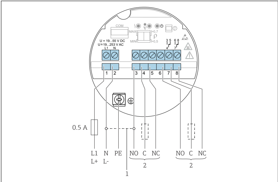
图 20 电子插件 FEL64: 通用电流连接型, 带继电器输出
