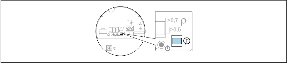
图 31 进行功能测试的按钮位置，适用电子插件 FEL61、FEL62、FEL64、FEL64DC、FEL67、FEL68
