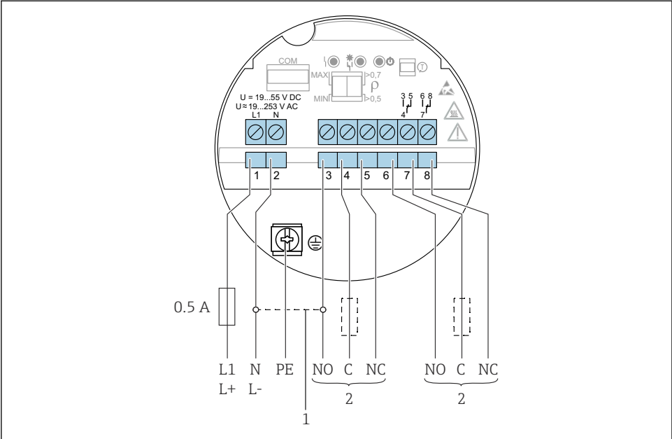
18 电子插件 FEL64: 通用电流连接型, 带继电器输出
