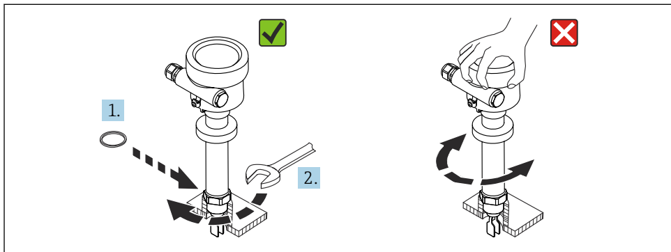
图 10 旋转拧入设备
