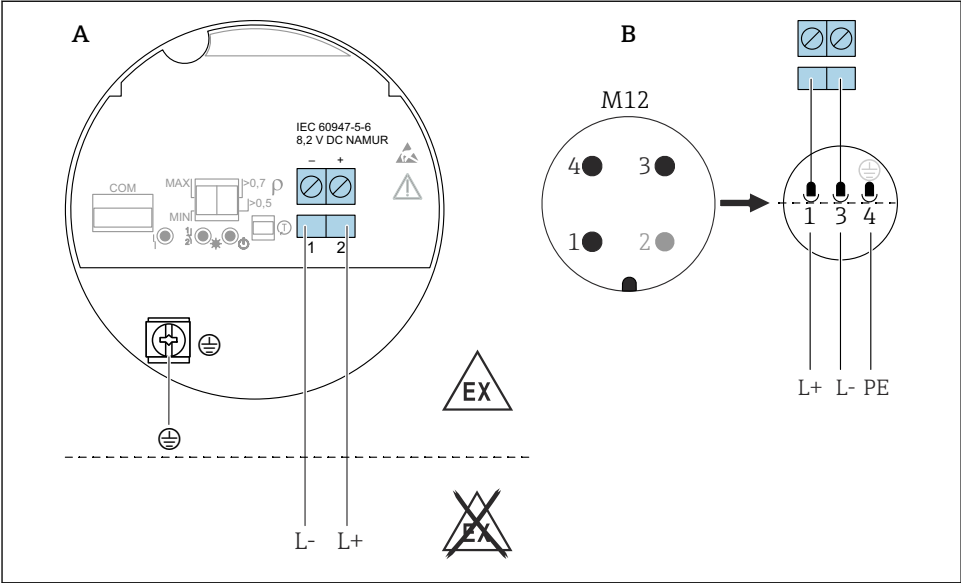
24 电子插件 FEL68: 两线制连接, NAMUR 信号 ( \geq 2.2 \text{ mA} / \leq 1.0 \text{ mA} )
