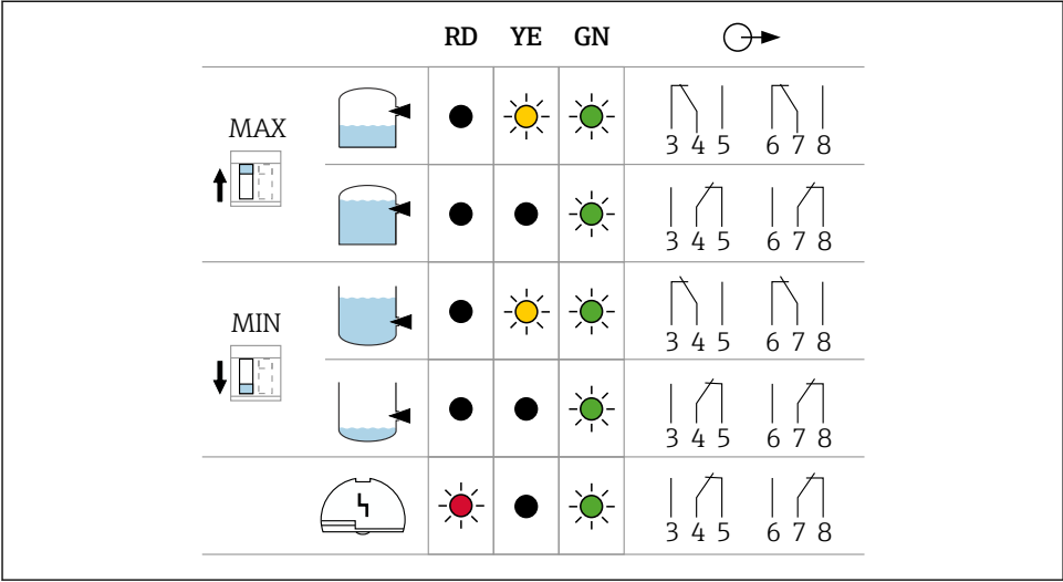
19 电子插件 FEL64 的继电器响应和故障信号
