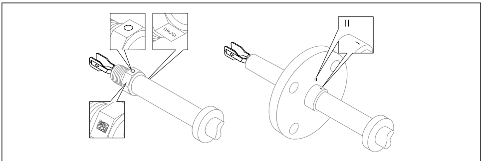
图 8 参照标记水平安装在罐体中时的音叉位置
