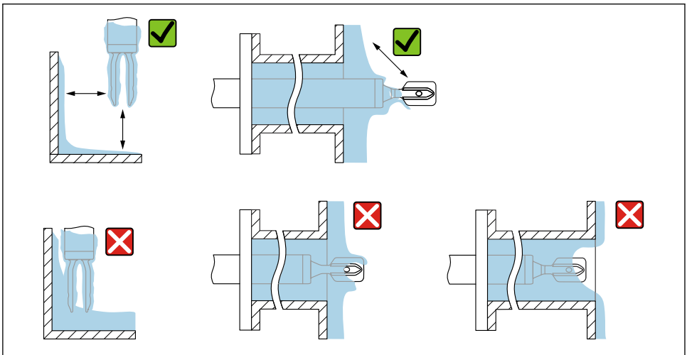
图 5 安装实例：测量高粘度过程介质
