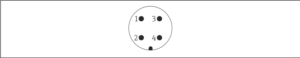
4 Rozmieszczenie styków w gnieździe przyłączeniowym 7/8"
