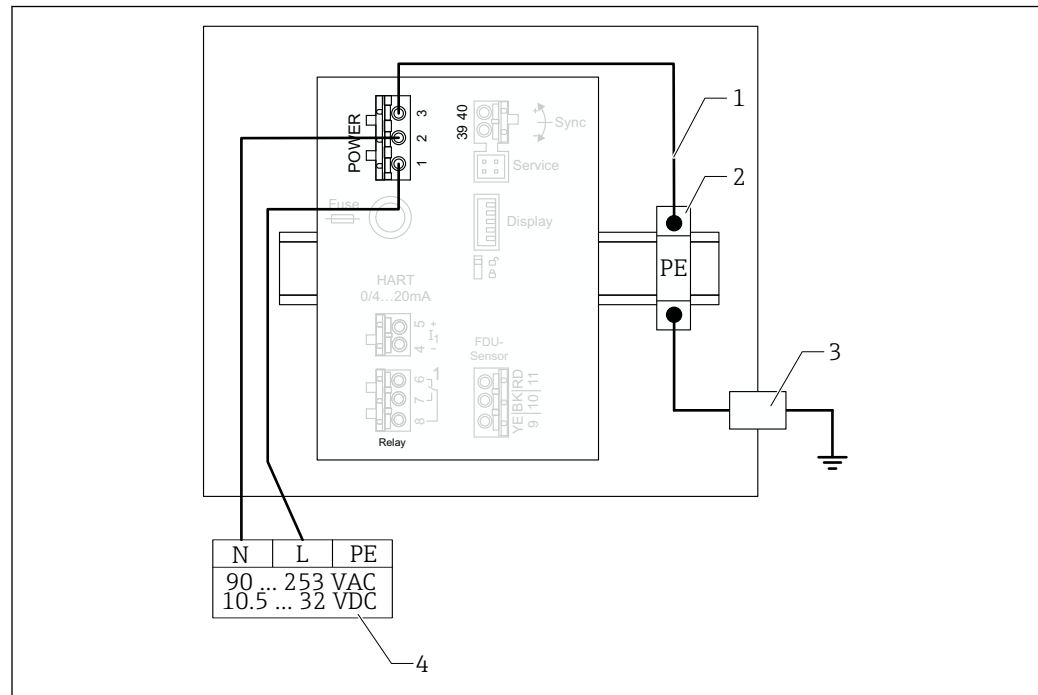
23 Conexión de la alimentación en la caja de aluminio para montaje en campo
