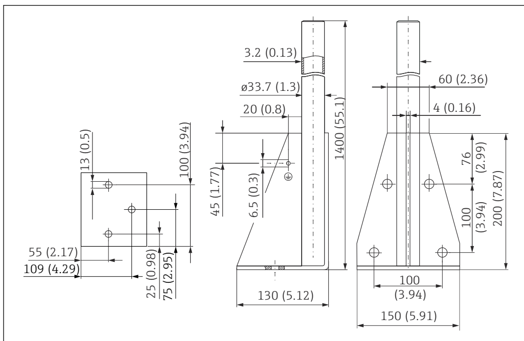
75 Medidas. Unidad de medida mm (in)
