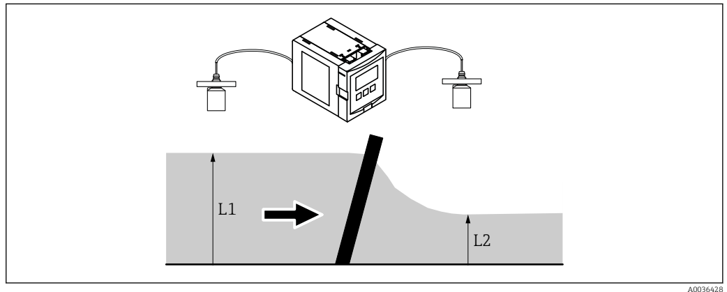
65 Principio de funcionamiento de la función de control de rejillas
