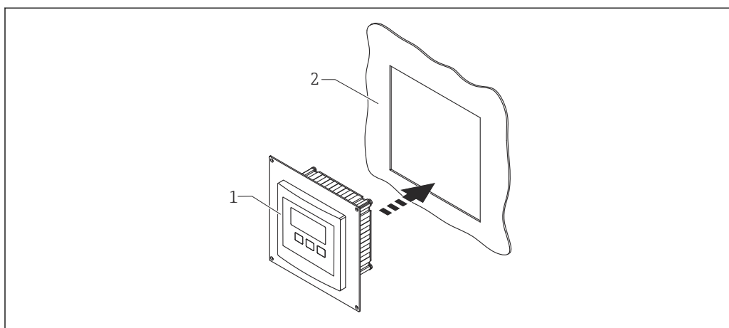
76 Uso de la placa adaptadora
