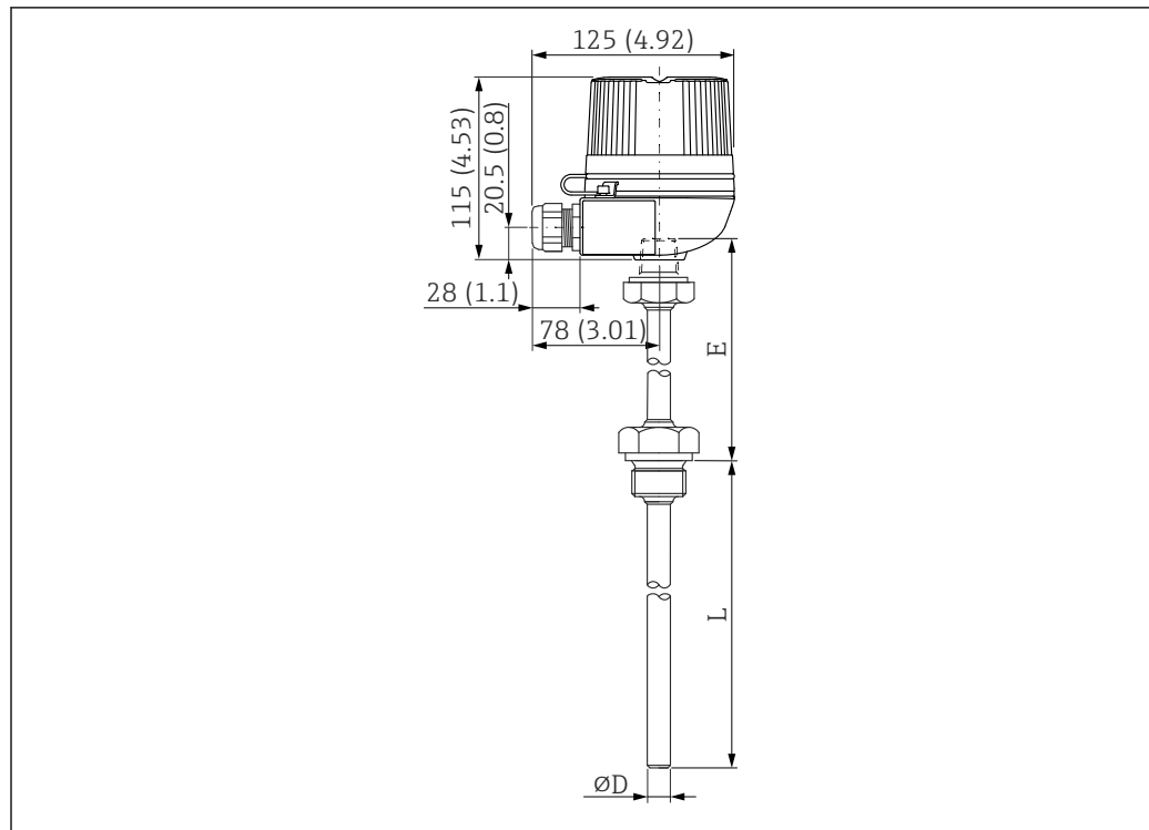
77 Estructura del Omnigrad S TR61; medidas: mm (in)
