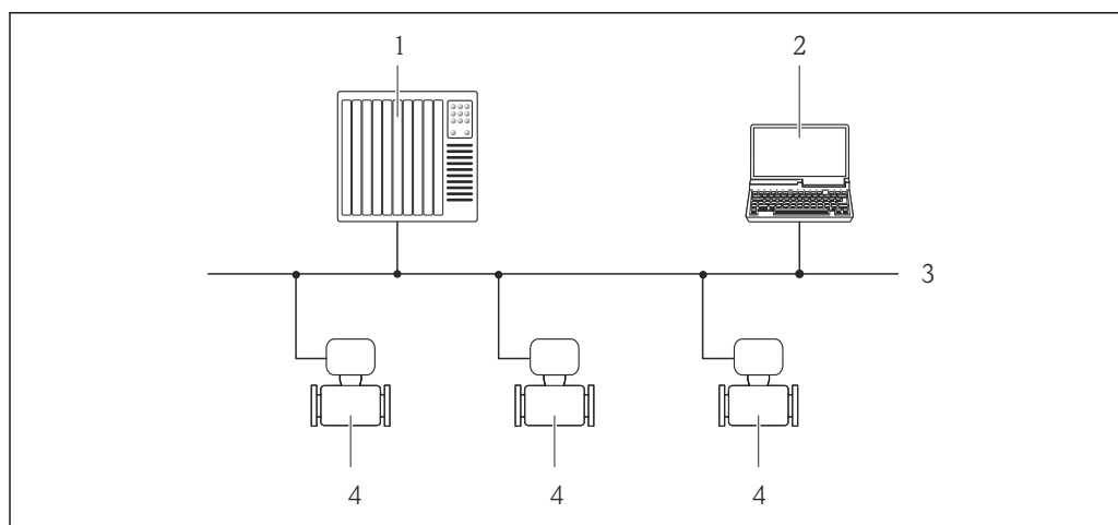
36 PROFIBUS DP ネットワークを介したリモート操作のオプション
