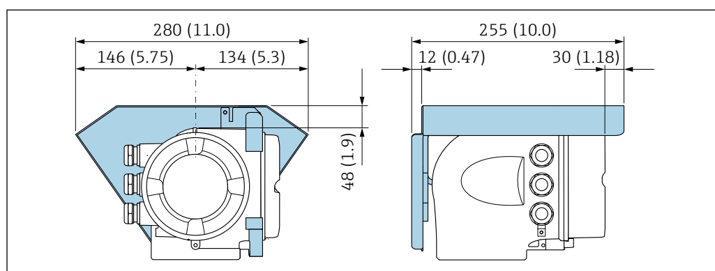
26 単位 mm (in)
