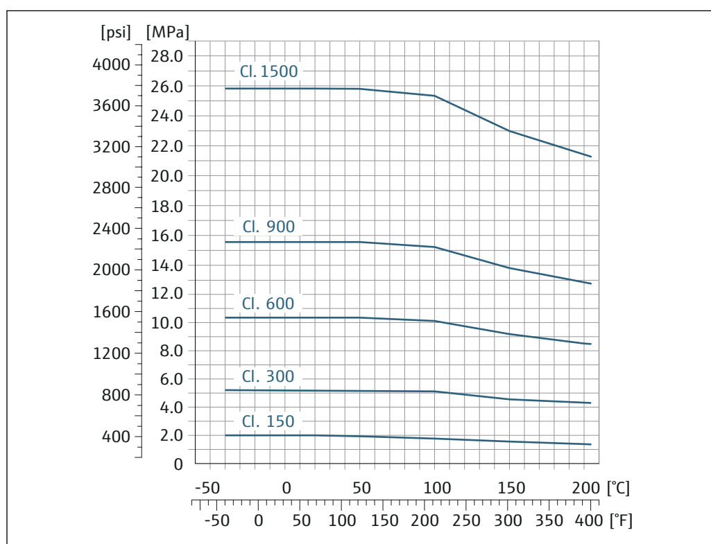
図 18 フランジ材質：ステンレス 1.4410/F53 25Cr 二相鋼（スーパー二相鋼）
