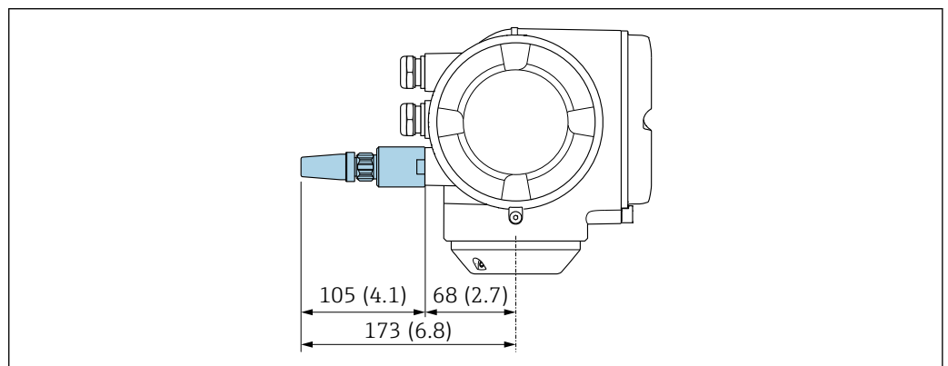
図 28 単位 mm (in)
