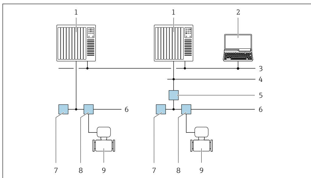
35 FOUNDATION Fieldbus ネットワークを介したリモート操作のオプション
