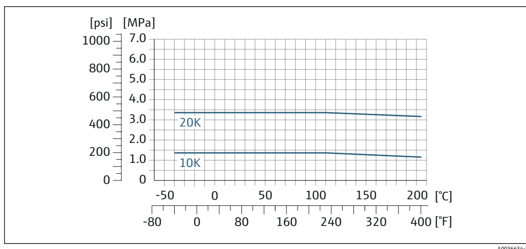
図 19 フランジ材質：ステンレス 1.4410/F53 25Cr 二相鋼（スーパー二相鋼）
