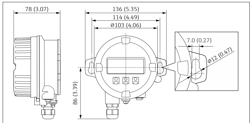
図 23 単位 mm (in)
