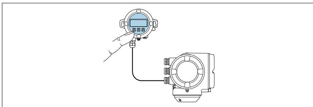
図 32 リモートディスプレイと操作モジュール DKX001 を使用した操作
