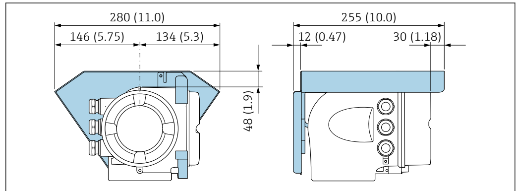
図 22 単位 mm (in)
