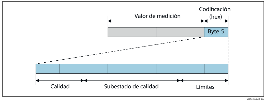
39 Estructura del byte de codificación
