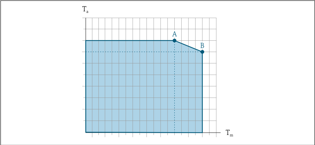
34 Rappresentazione esemplificativa, valori nella tabella sottostante. T_a Temperatura ambiente T_m Temperatura del fluido A Temperatura del fluido massima consentita T_m con T_{a\max} = 60\text{ °C} (140 °F); temperature del fluido superiori T_m richiedono una temperatura ambiente ridotta T_a B Temperatura ambiente massima consentita T_a per la temperatura del fluido massima specificata T_m del sensore
