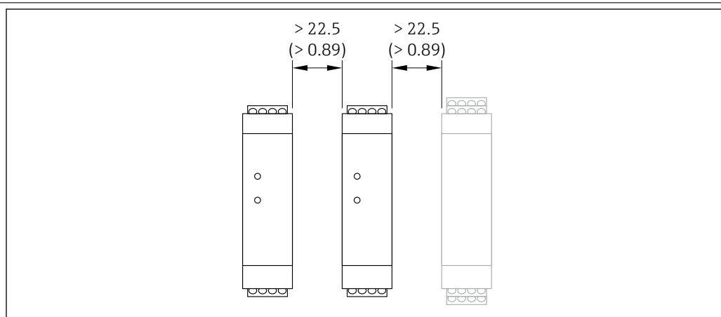
図 13 追加の Promass 100 安全バリアまたはその他のモジュールとの最小距離。単位 mm (in)
