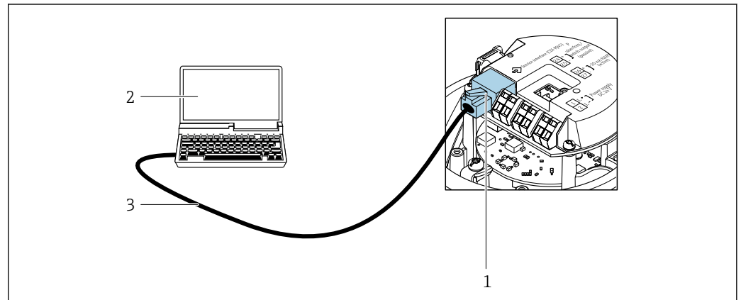
図 30 「出力」のオーダーコードの接続、オプション B : 4~20 mA HART、パルス/周波数/スイッチ出力
