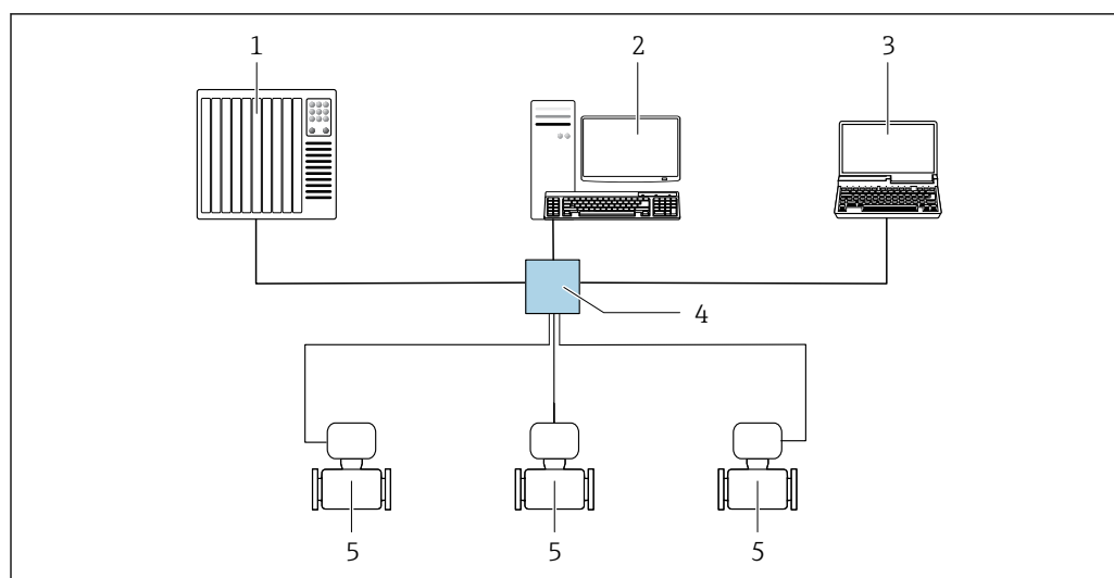
図 28 EtherNet/IP ネットワーク経由のリモート操作オプション：スター型トポロジー
