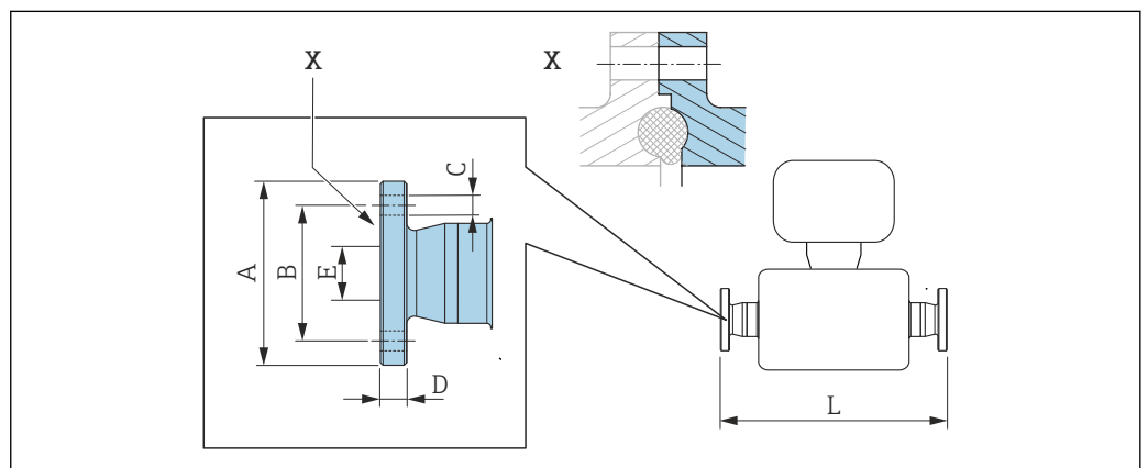
図 24 X の詳細 : 非対称型プロセス接続 ; 着色部分が供給されます。
