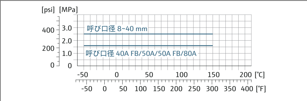
図 18 フランジ材質 グレード 2 チタン
