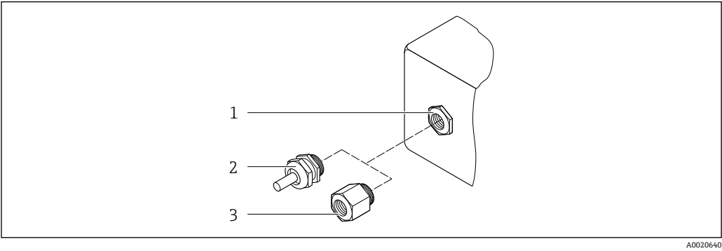
図 25 可能な電線口/ケーブルグランド
