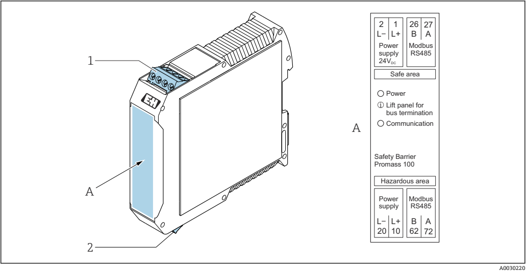
8 Promass 100 安全バリア、端子付き 1 非危険場所：ゾーン 2、Class I、Division 2 2 本質安全区域
