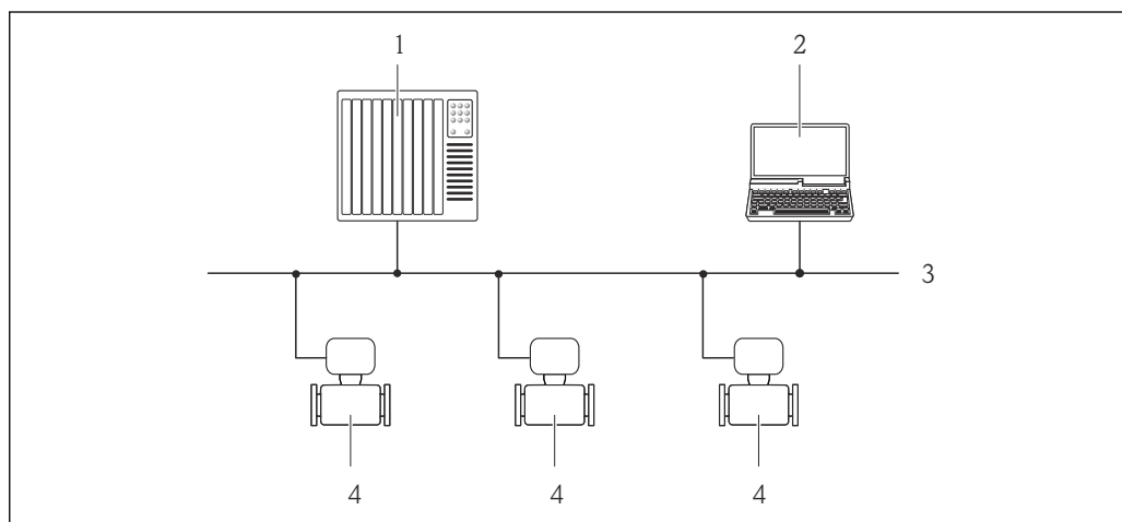
図 27 PROFIBUS DP ネットワークを介したリモート操作のオプション
