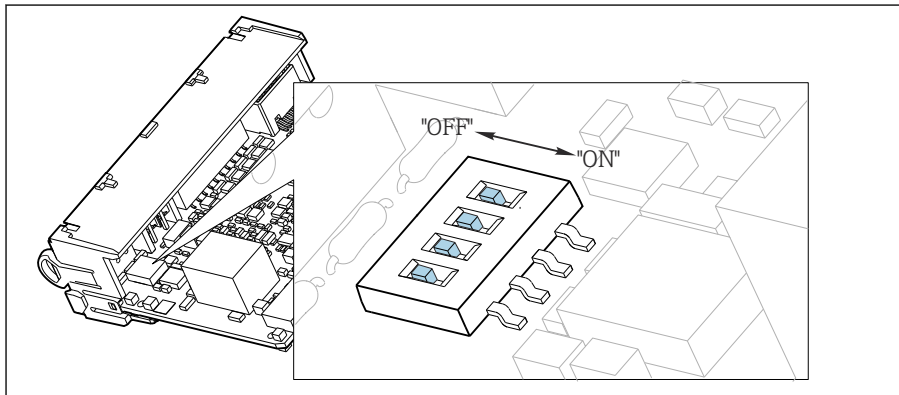
31 Comutatorul de tip DIP switch pentru terminație internă
