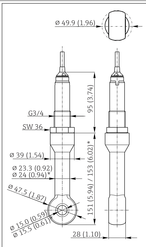
16 Versão com rosca G \frac{3}{4} . Unidade de medida mm (in)
