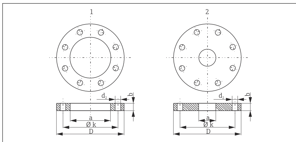
19 Dimensões do flange
