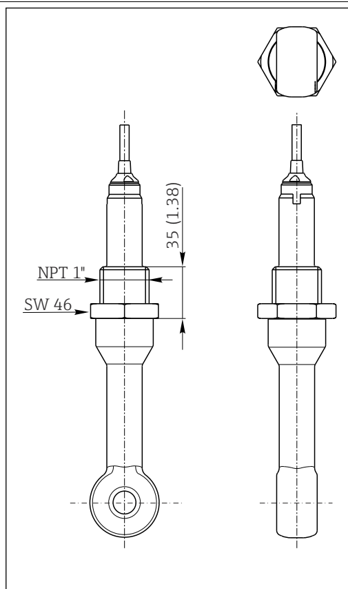
17 Versão, rosca NPT 1". Unidade de medida mm (in)
