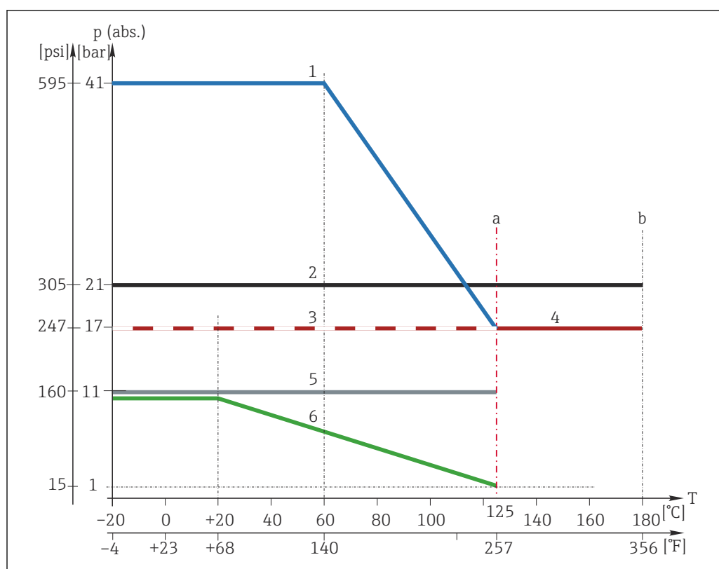
14 Curvas de temperatura/pressão
