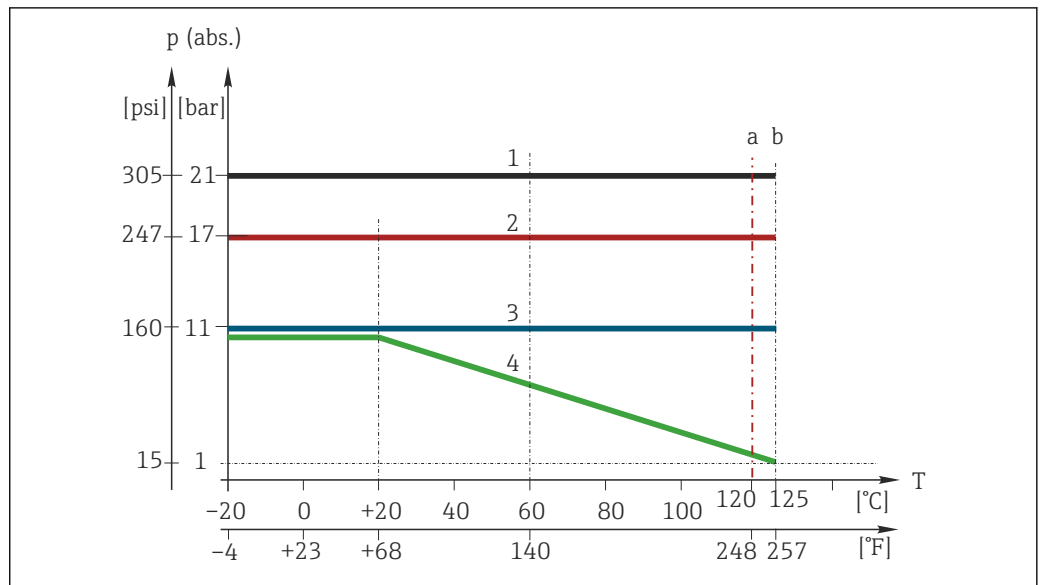
12 Curvas de temperatura/pressão
