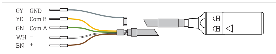
12 Mätkabel CYK10 /CYK20
