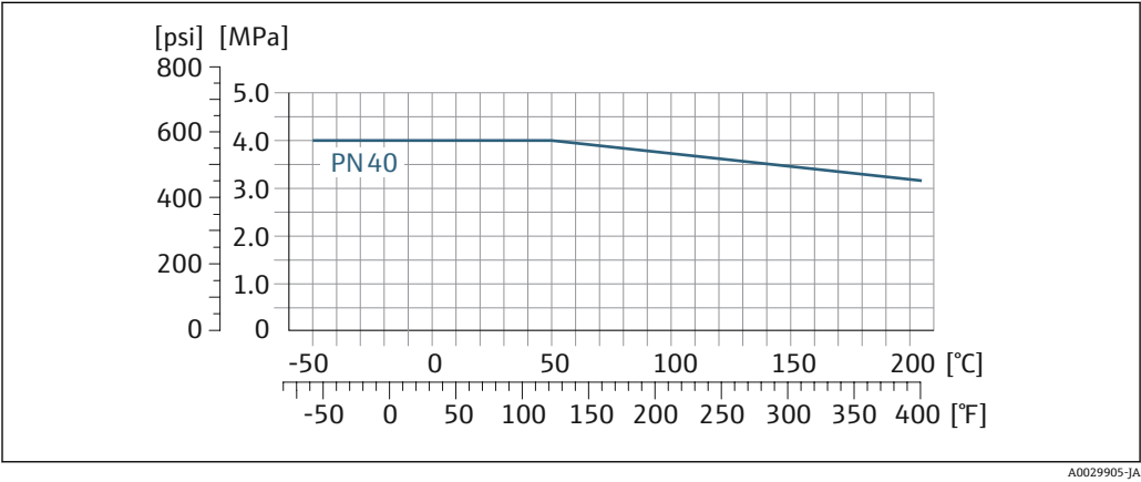
図 17 フランジ材質 1.4404 (SUS F316 相当または SUS F316L 相当)
