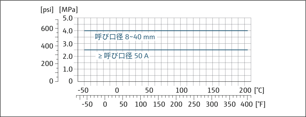
図 22 接続部の材質 1.4435 (SUS 316L 相当)
