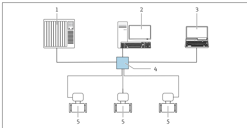
図 50 EtherNet/IP ネットワーク経由のリモート操作オプション：スター型トポロジー
