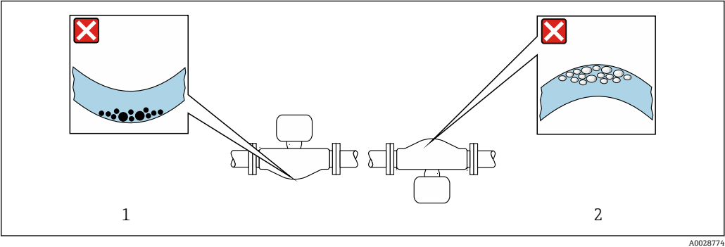
図 14 弓形計測チューブセンサの取付方向
