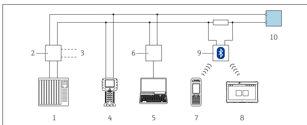
図 43 HART プロトコル経由のリモート操作用オプション（パッシブ）
