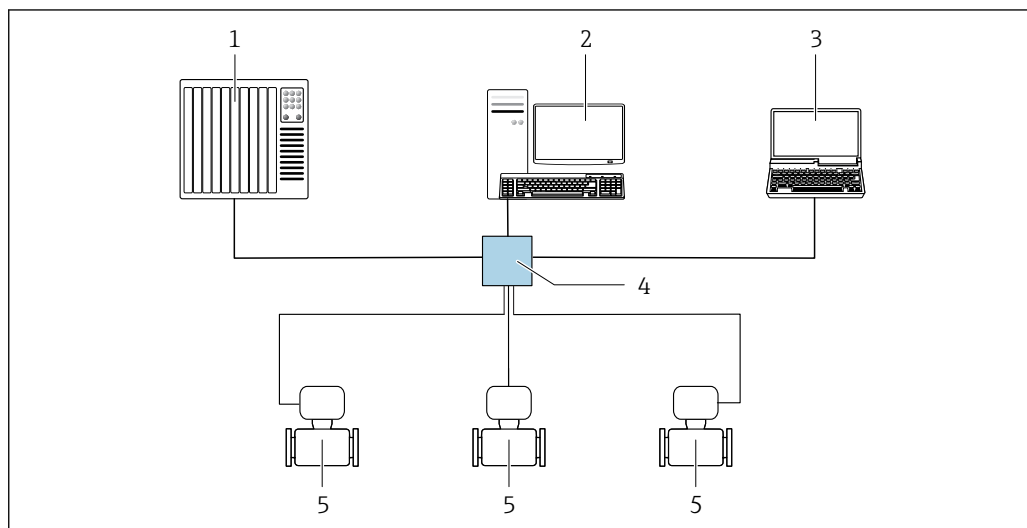
図 49 Modbus TCP over Ethernet - 100 Mbit/s 経由のリモート操作用オプション：スター型トポロジー
