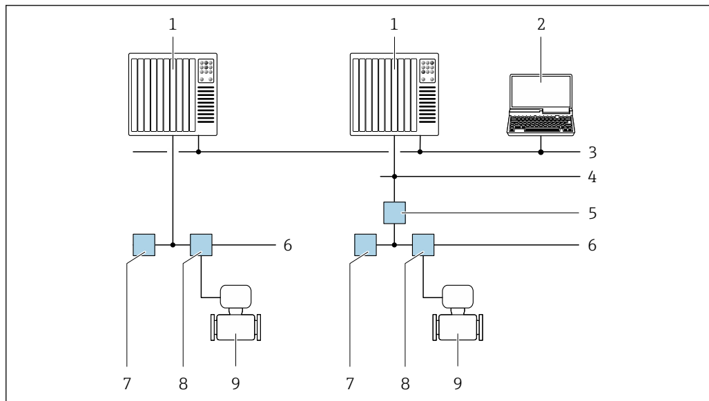
図 44 FOUNDATION Fieldbus ネットワークを介したリモート操作のオプション
