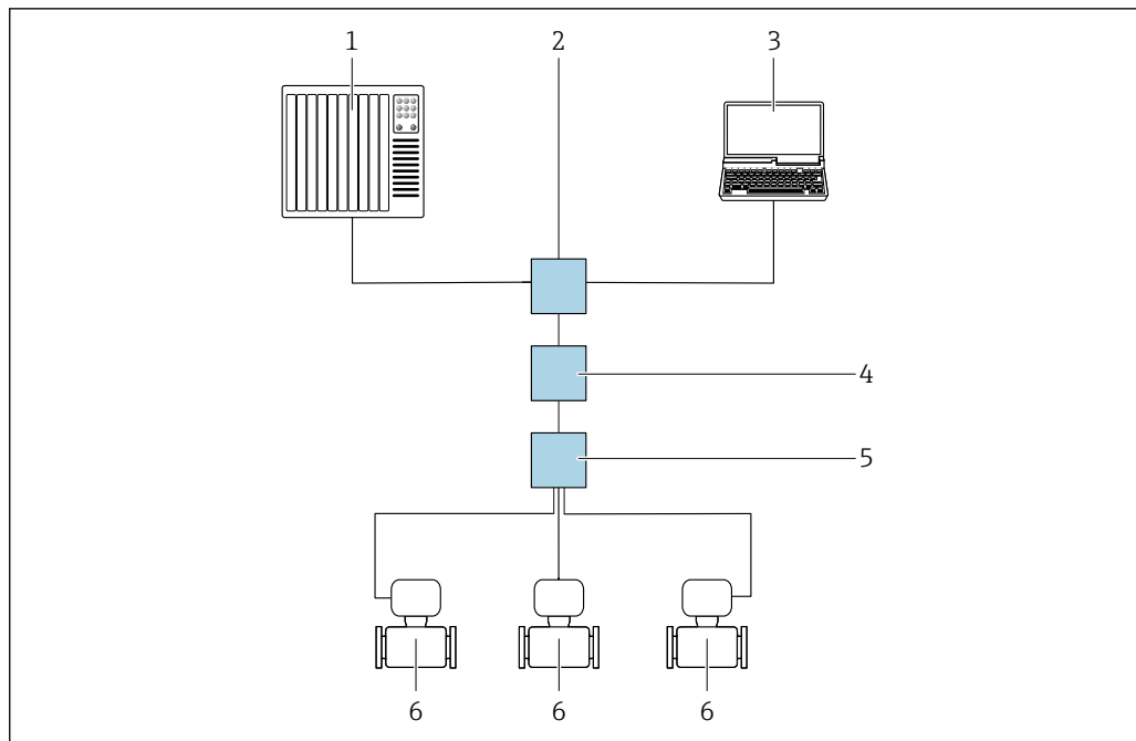
図 48 Modbus TCP over Ethernet-APL プロトコル経由のリモート操作用オプション（アクティブ）
