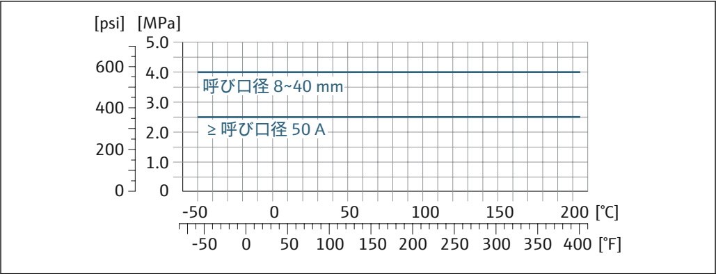
図 21 フランジ材質 1.4435 (SUS 316L 相当)
