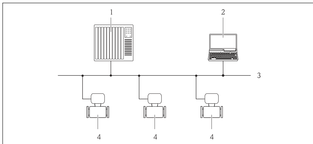
図 45 PROFIBUS DP ネットワークを介したリモート操作のオプション
