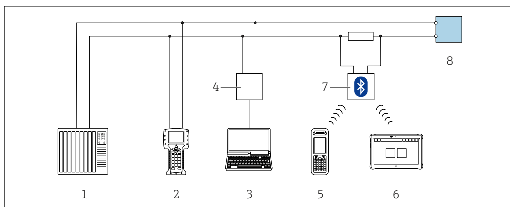
図 42 HART プロトコル経由のリモート操作用オプション（アクティブ）
