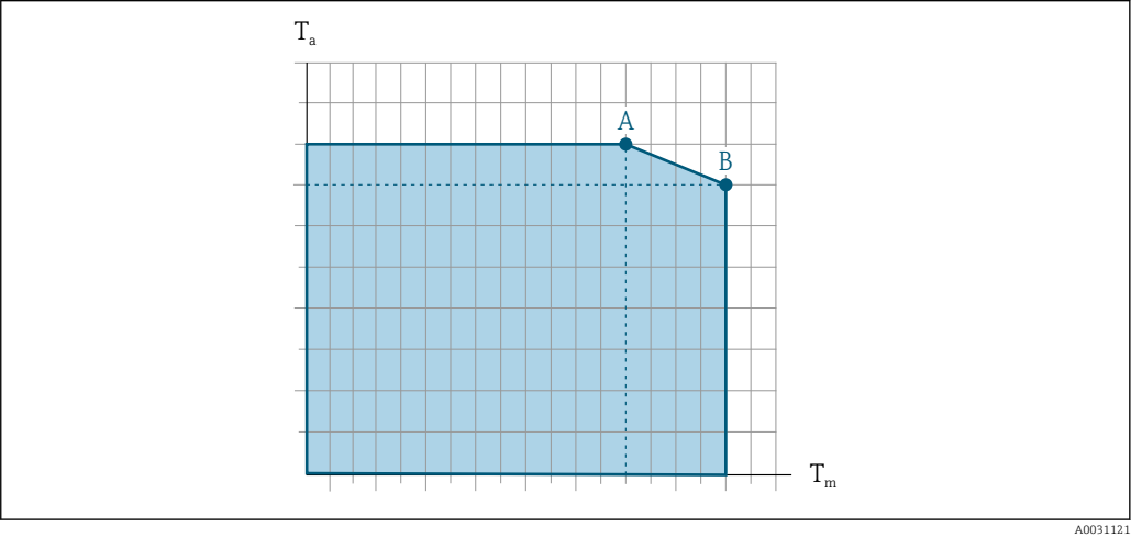
33 Representação exemplar, valores na tabela abaixo. T_a Temperatura ambiente T_m Temperatura do meio A Temperatura máxima permitida do meio T_m a T_a máx. = 60\text{ °C (140 °F)} ; temperaturas do meio mais altas T_m requerem uma redução na temperatura ambiente T_a B Temperatura ambiente T_a máxima permitida para a temperatura média T_m máxima especificada do sensor
