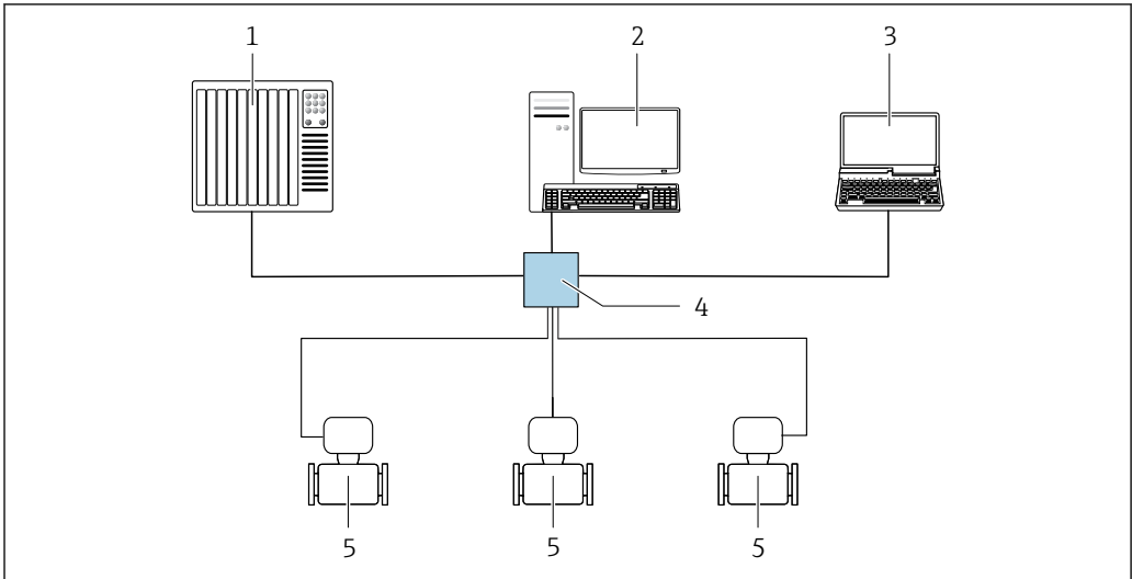
图 25 通过 Modbus TCP + Ethernet 进行远程操作 - 100 Mbit/s: 星形拓扑结构
