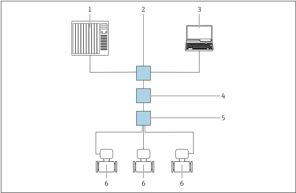
图 24 通过 Modbus TCP + Ethernet-APL 通信进行远程操作（有源信号）
