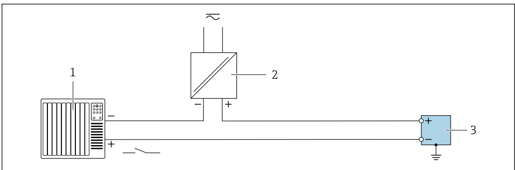
17 状态输入 1 自动化系统，带无源开关量输出（例如 PLC） 2 电源 3 变送器，带状态输入
