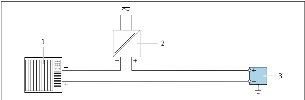
16 接线实例：继电器输出 1 自动化系统，带开关量输入（例如 PLC） 2 电源 3 变送器，带继电器输出
