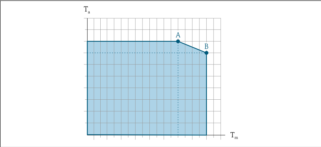
33 示例图，具体数值见下表。 T a 环境温度 T m 介质温度 A 介质温度 T m 越高 (T a max = 60 °C (140 °F) 时)，所需的环境温度 T a 越低 B 传感器最高允许介质温度 T m 对应的最高允许环境温度 T a
