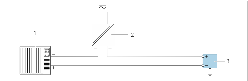
15 接线实例：脉冲输出/频率输出/开关量输出（无源） 1 自动化系统，带脉冲输入/频率输入/开关量输入（例如 PLC） 2 电源 3 变送器，带脉冲输出/频率输出/开关量输出（无源）
