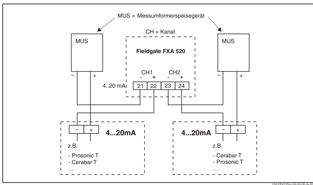
Abb. 7: Klemmenbelegung für Anschluss mit Messumformerspeisegerät
