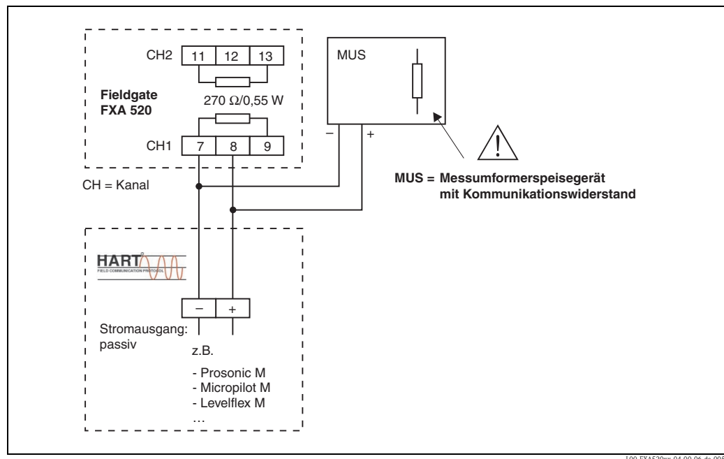
Abb. 3: Klemmenbelegung für Anschluss mit Messumformerspeisegerät mit Kommunikationswiderstand
