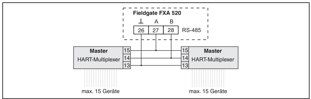
Abb. 8: Klemmenbelegung für Anschluss mit HART-Multiplexer (Master/Master)
