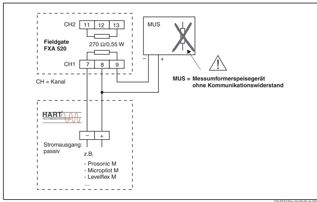
Abb. 4: Klemmenbelegung für Anschluss mit Messumformerspeisegerät ohne Kommunikationswiderstand
