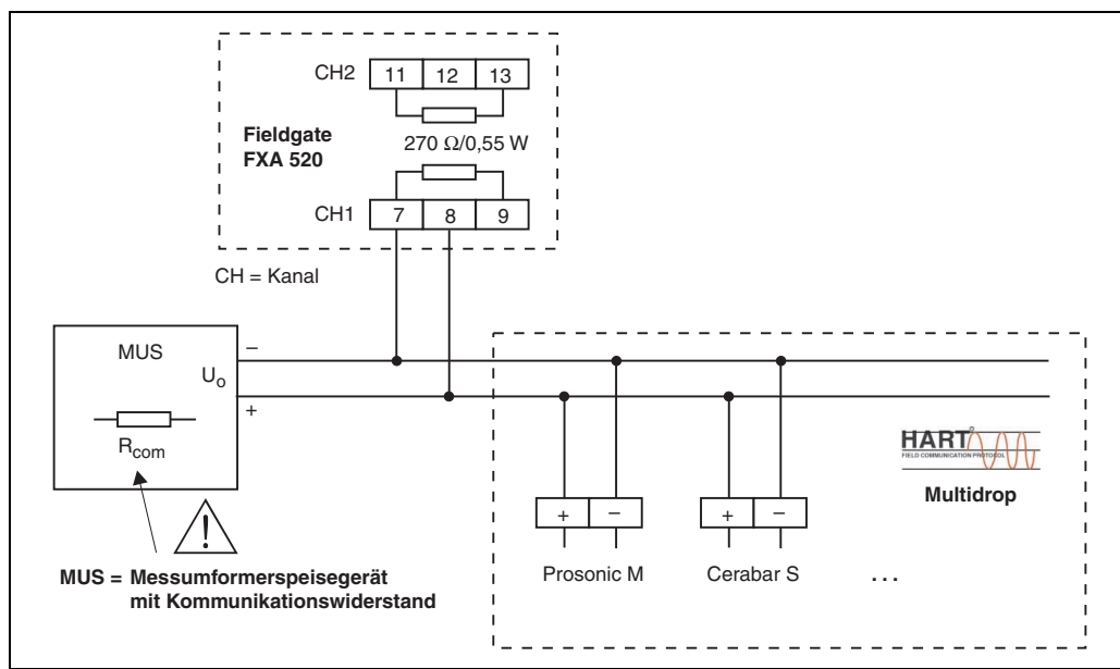
Abb. 6: Klemmenbelegung für Anschluss mit Messumformerspeisegerät ( mit Kommunikationswiderstand) im Multidrop-Betrieb
