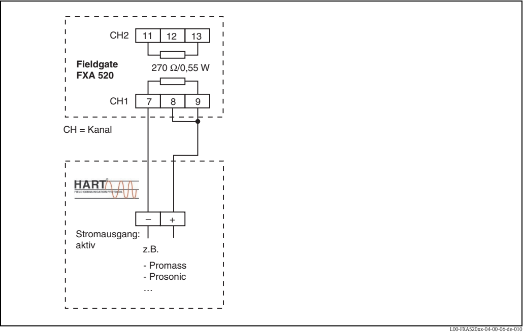
Abb. 5: Klemmenbelegung für Anschluss mit aktivem Stromausgang
