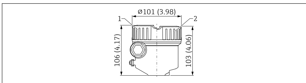
26 Dimensioni della custodia a vano unico, in alluminio, rivestita. Unità di misura mm (in)
