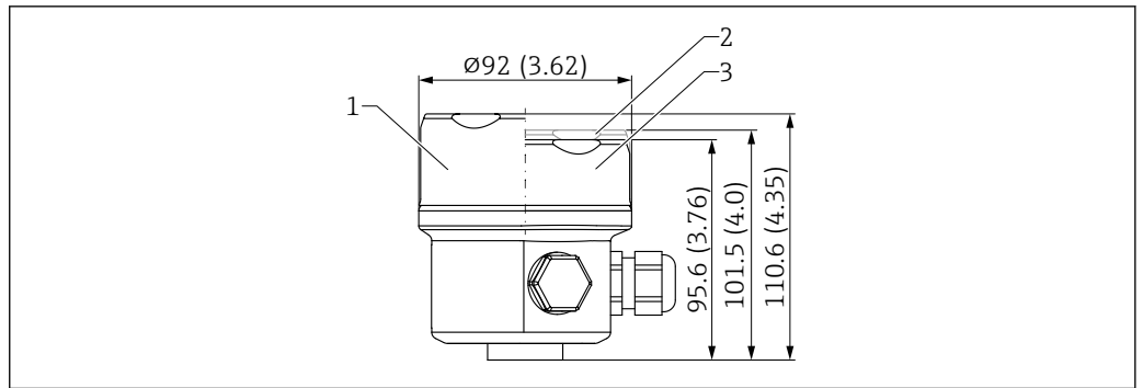
28 Dimensioni della custodia a vano unico, 316L, igienica. Unità di misura mm (in)
