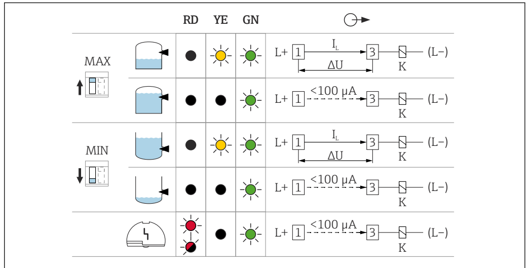
3 Commutazione FEL42, segnalazione tramite LED
