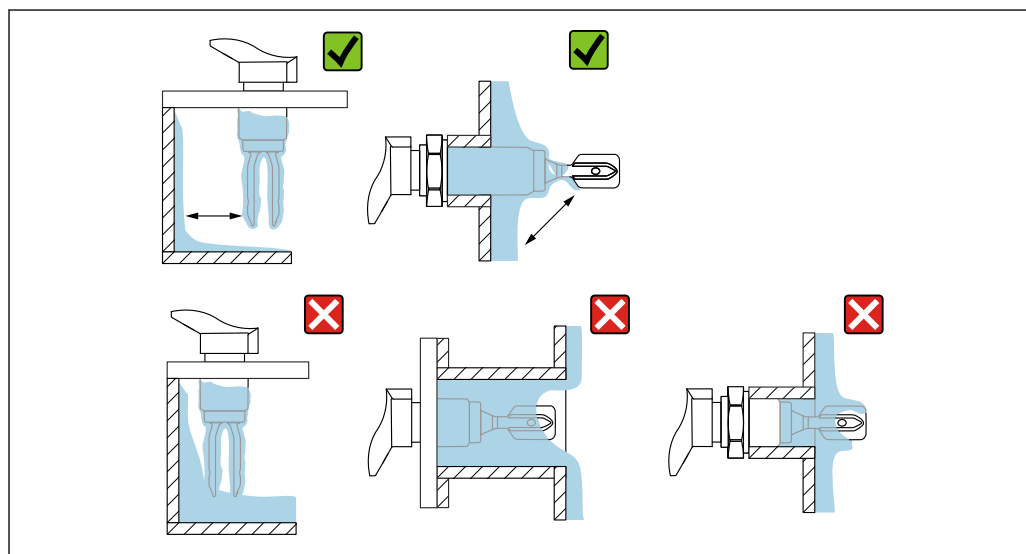
13 Esempi di installazione per un fluido di processo estremamente viscoso
