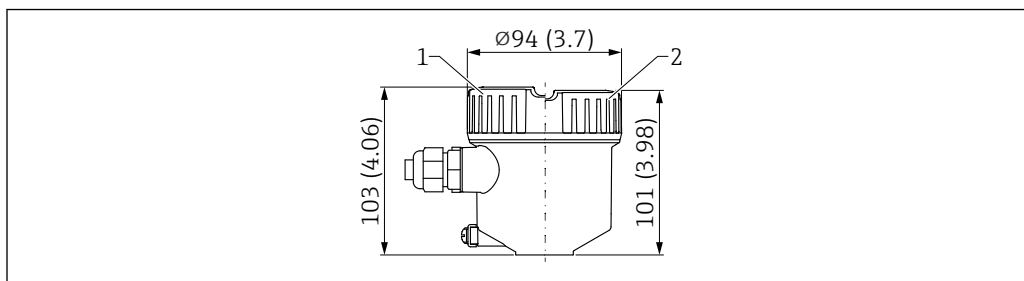
25 Dimensioni della custodia a vano unico, in plastica. Unità di misura mm (in)
