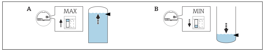
45 Posizione di commutazione sull'inserto elettronico per modalità di sicurezza MAX/MIN
