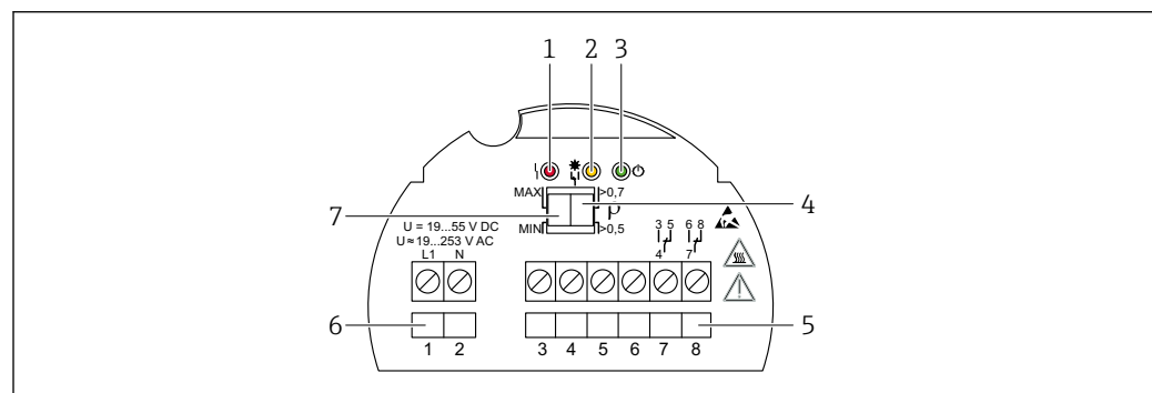
44 Esempio di inserto elettronico FEL44
