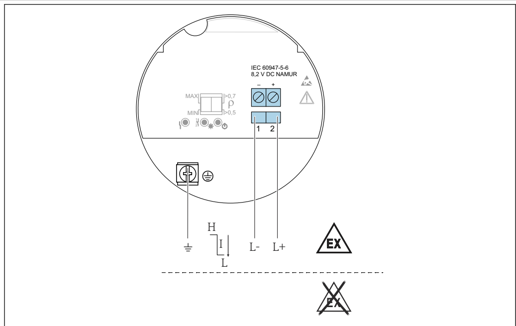
6 NAMUR a due fili >2,2 mA/≤ 1,0 mA, inserto elettronico FEL48
