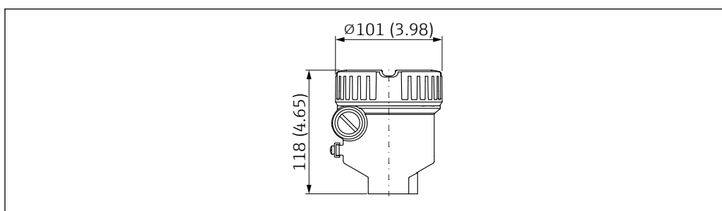
27 Dimensioni della custodia a vano unico, in alluminio, rivestita (Ex d/XP), coperchio senza vetro di ispezione. Unità di misura mm (in)
