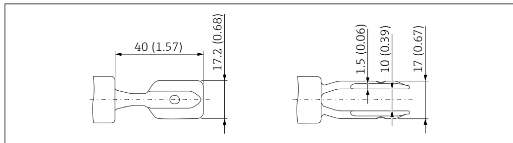
31 Diapason. Unità di misura mm (in)
