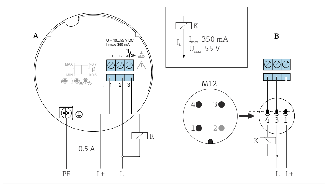
2 Assegnazione morsetti FEL42
