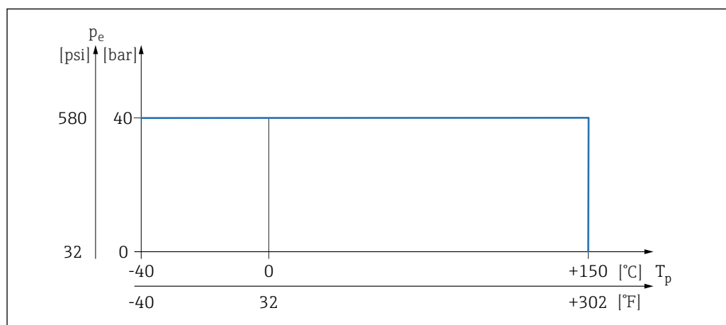
23 Temperatura di processo FTL41
