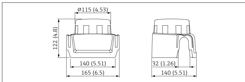
47 Dimensioni del tettuccio di protezione dalle intemperie, plastica, XW111. Unità di misura mm (in)
