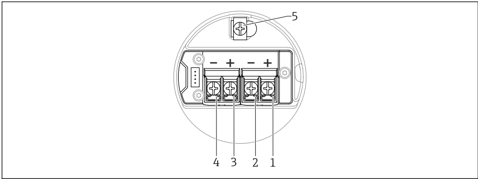
14 Affectation des bornes dans le compartiment de raccordement ; 4 ... 20 mA HART, sortie tout ou rien ; boîtier à double compartiment, forme L
