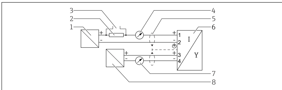
7 Diagramme fonctionnel 4 ... 20 mA HART + 4 ... 20 mA analogique
