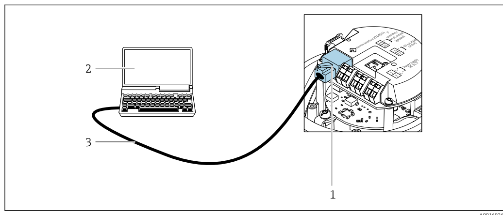
14 Raccordement pour caractéristique de commande "Sortie", Option B : 4-20 mA HART, sortie impulsion/fréquence/tor
