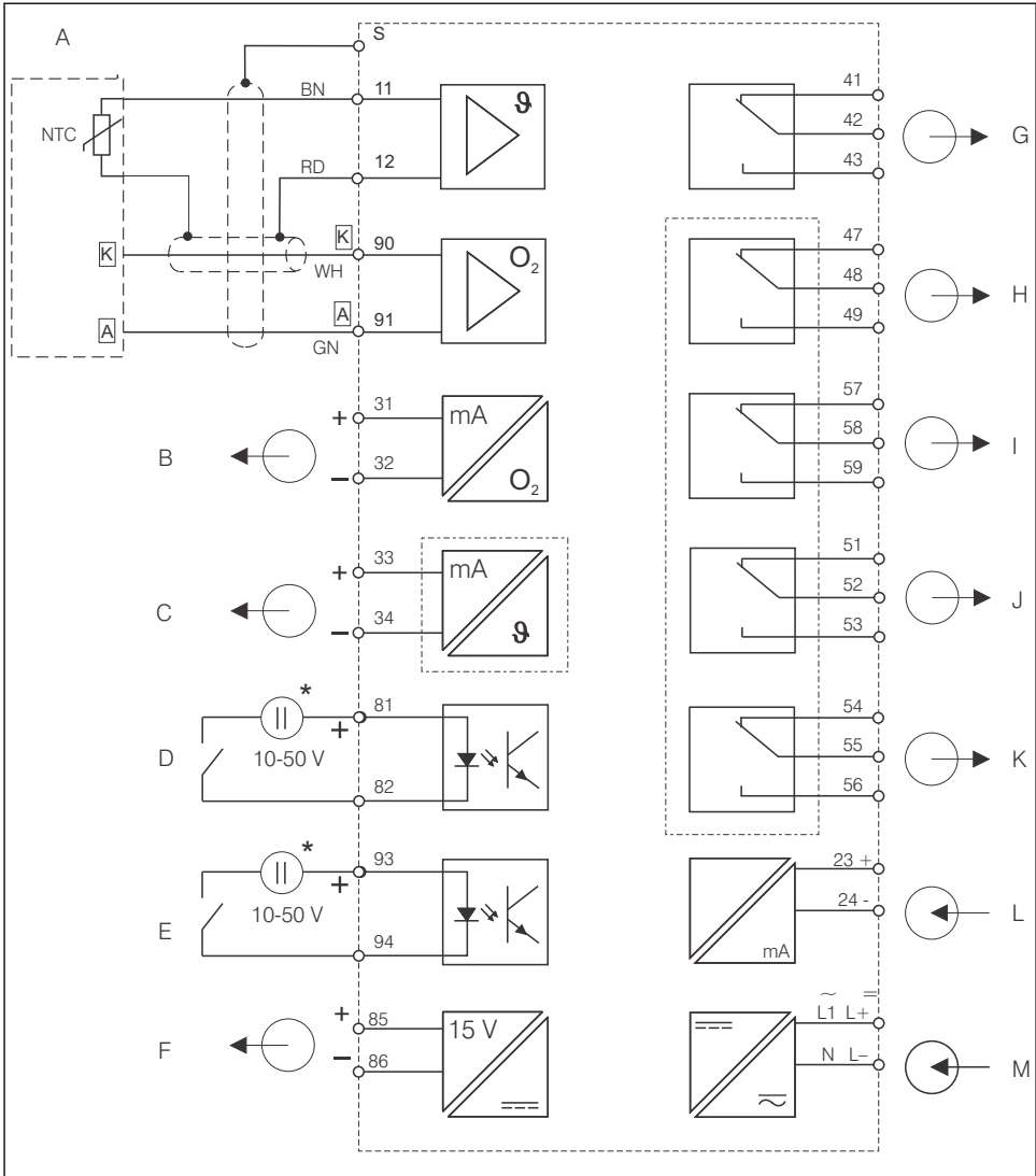
3 트랜스미터 전기 연결, DX 또는 DS 버전
