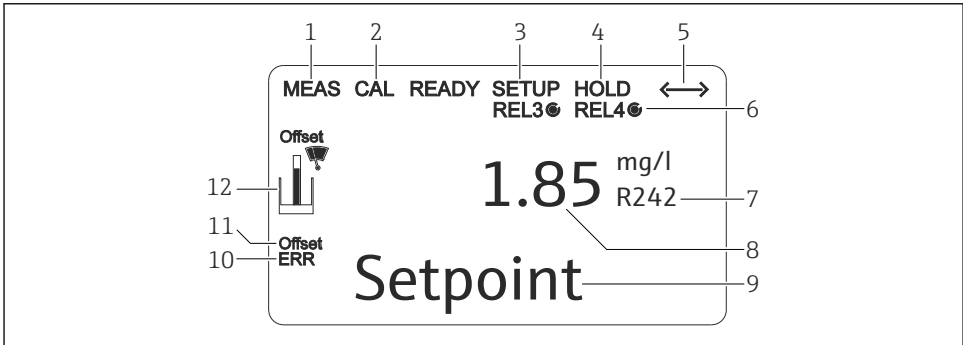
☞ 11 트랜스미터 LC 디스플레이
