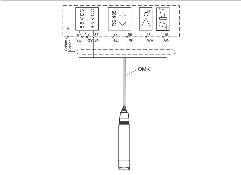
☒ 9 연결 예: COS31/71 및 OMK 케이블
