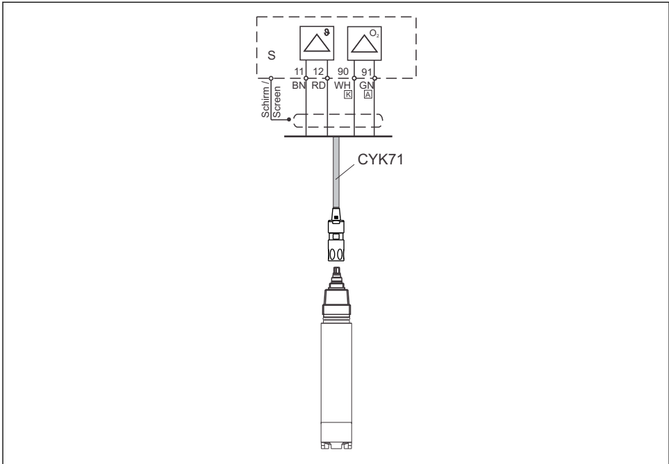
☞ 5 연결 예: COS41 및 CYK71 케이블
