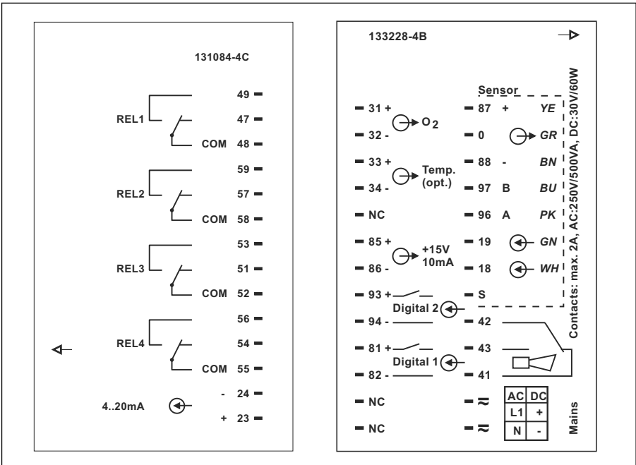
☞ 7 Liquisys M 패널 설치 계기의 연결부 스티커, 버전 WX/WS
