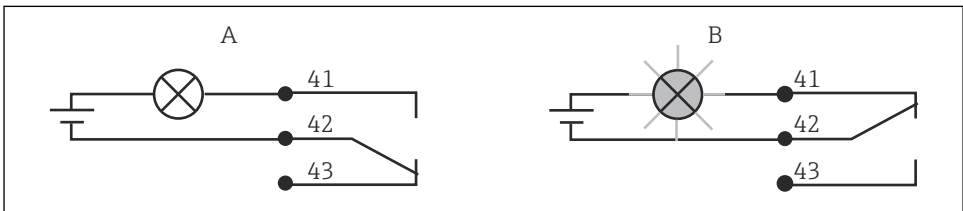
☒ 10 알람 접점에서 권장하는 이중 안전(fail-safe) 전환
