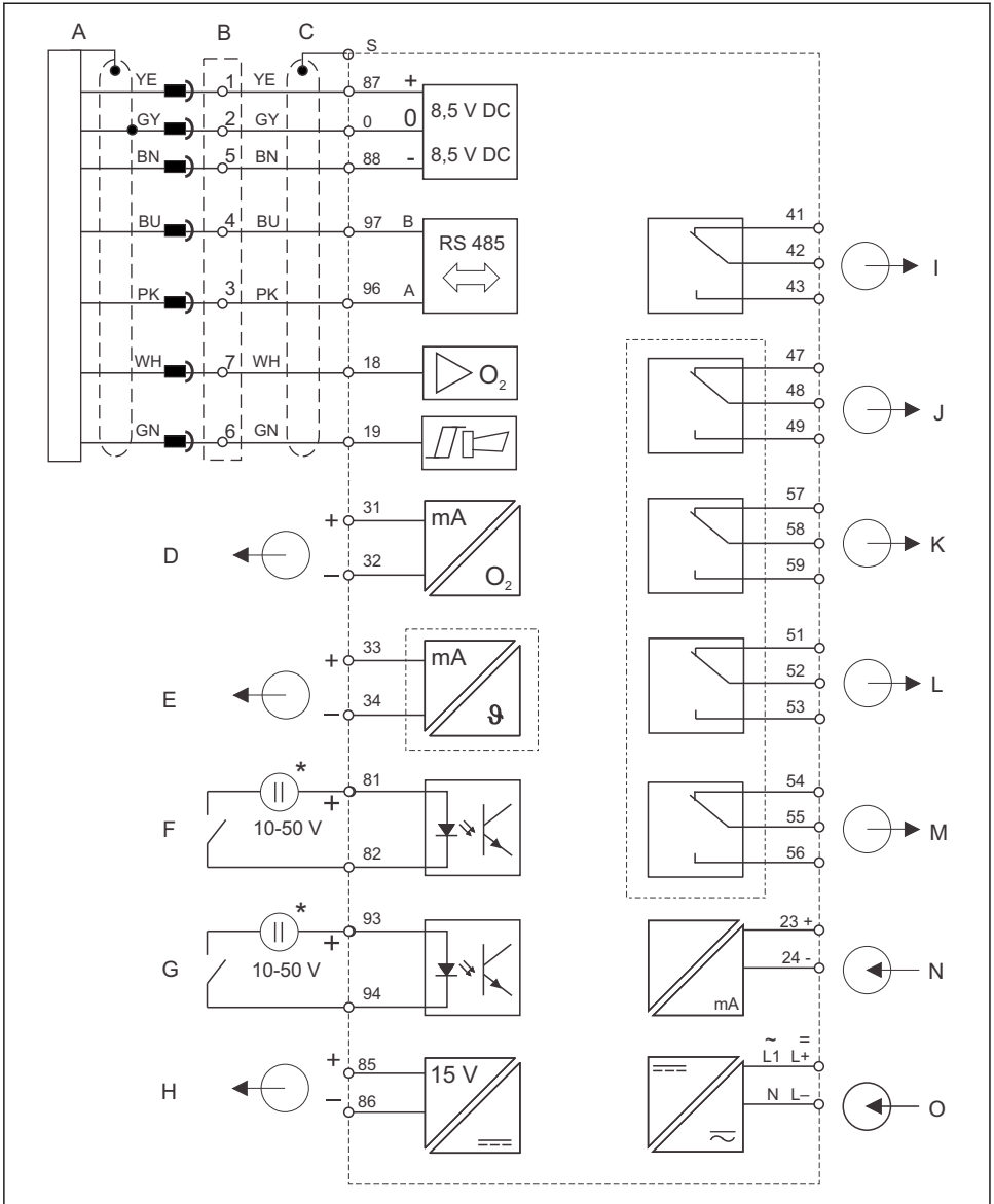
6 WX 또는 WS 버전의 Liquisys M COM223/253 전기 연결
