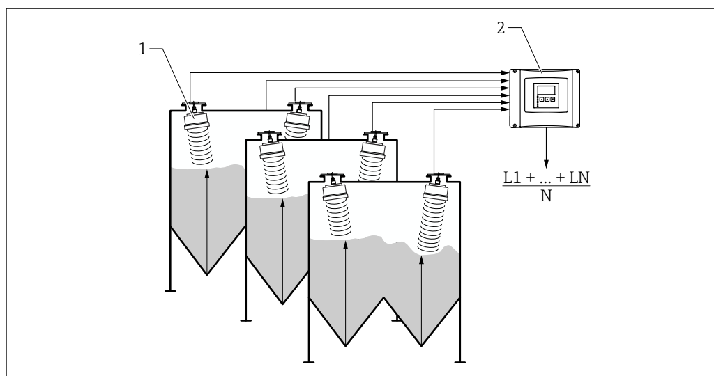
3 Mesure de niveau multivoie avec calcul de la moyenne
