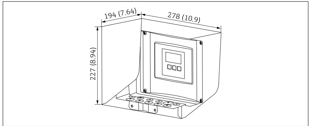
12 Capot de protection climatique pour boîtier de terrain en polycarbonate. Unité de mesure mm (in)
