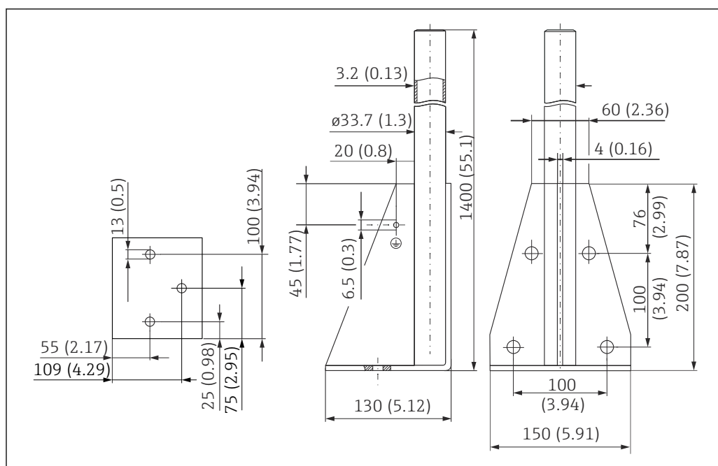
15 Dimensions. Unité de mesure mm (in)
