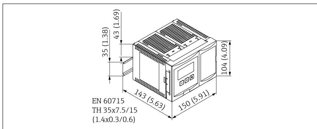
6 Dimensions du boîtier pour rail DIN ; dimensions en mm (in)
