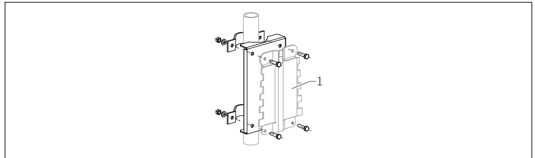
13 Plaque de montage pour boîtier de terrain en polycarbonate
