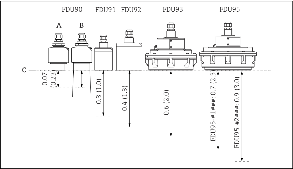
1 Distance de blocage des capteur à ultrasons FDU9x. Unité de mesure m (ft) A FDU90 sans tube de protection antidébordement B FDU90 avec tube de protection antidébordement C Point de référence de la mesure
