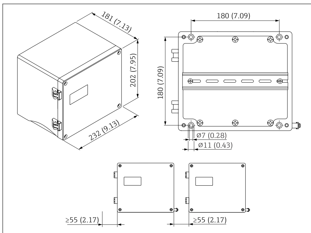
5 Dimensions du Prosonic S avec boîtier de terrain en aluminium. Unité de mesure mm (in)
