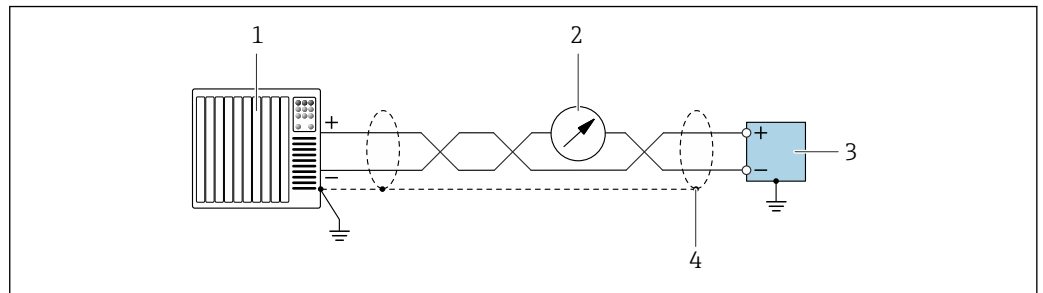
25 Exemple de raccordement pour sortie courant 4 ... 20 mA avec HART (active)
