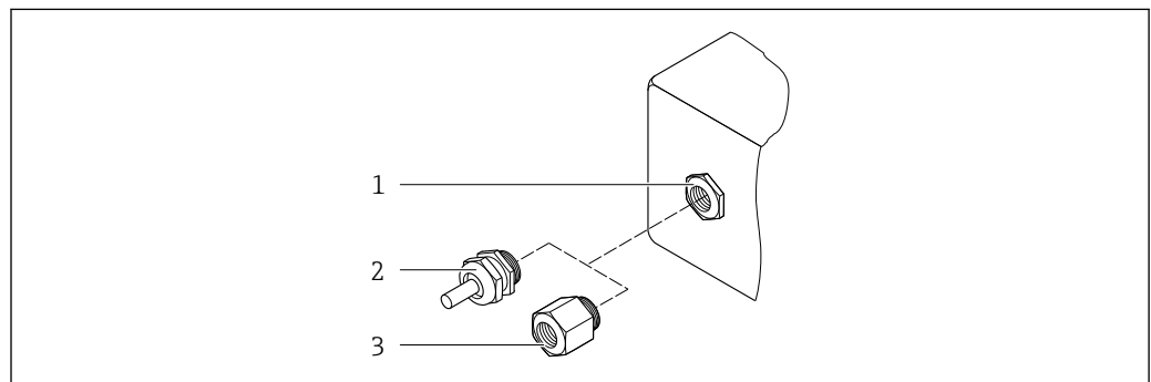
45 Entrées de câble/presse-étoupe possibles
