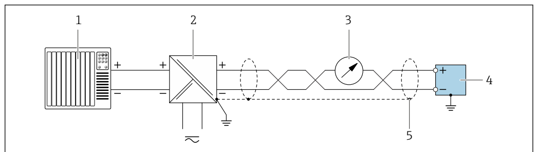
26 Exemple de raccordement pour sortie courant 4 ... 20 mA avec HART (passive)
