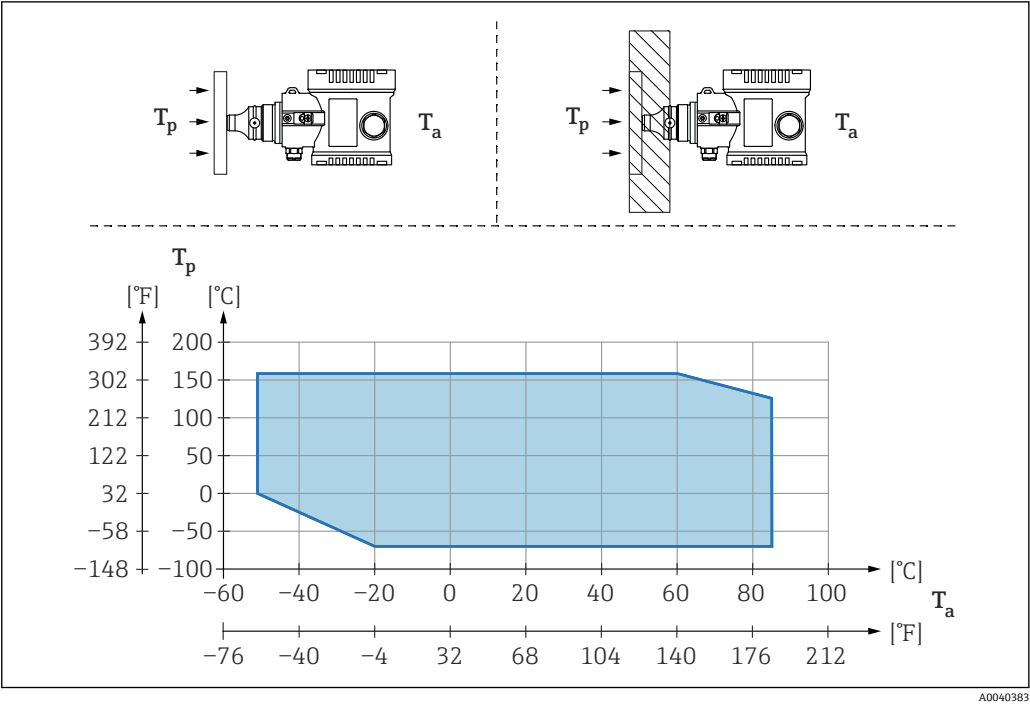
安装带直连型隔膜密封系统的仪表
