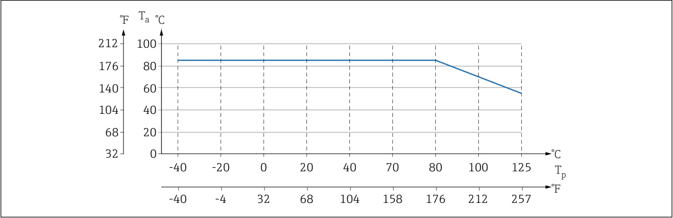
图 6 以上为无保温层竖直安装时的温度范围。
