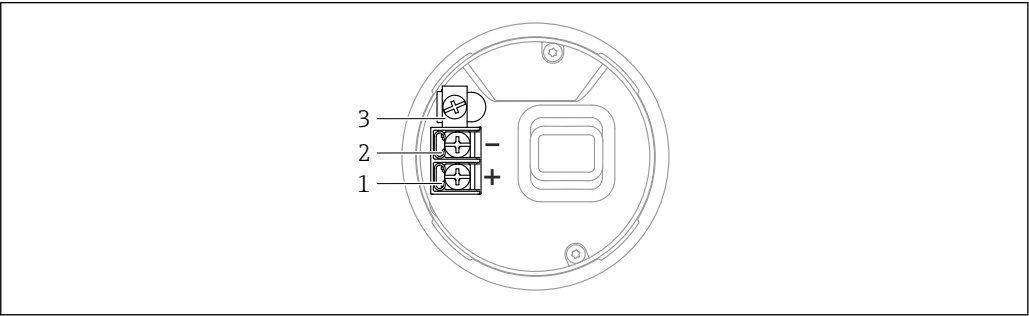
图 2 接线腔中的接线端子和接地端
