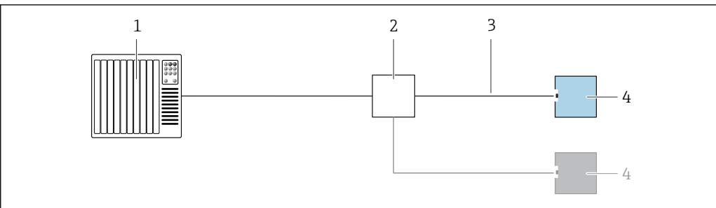
5 接线示例: PROFINET + Ethernet-APL
