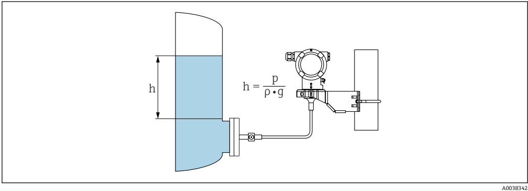
图 1 示意图：带毛细管隔膜密封系统的仪表
