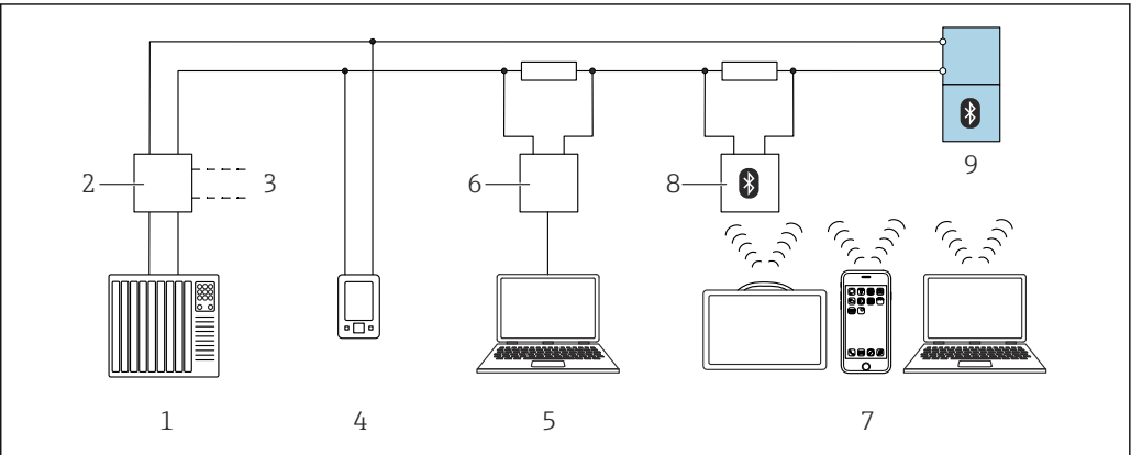
图 9 通过 HART 通信进行远程操作
