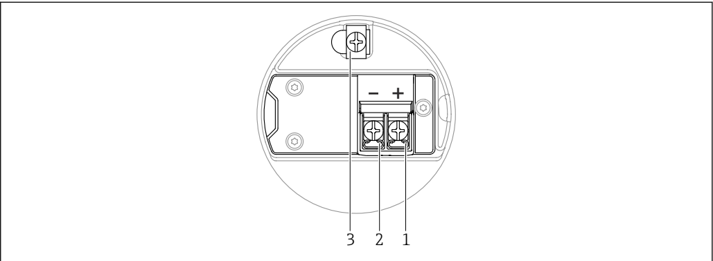
图 3 接线腔中的接线端子和接地端
