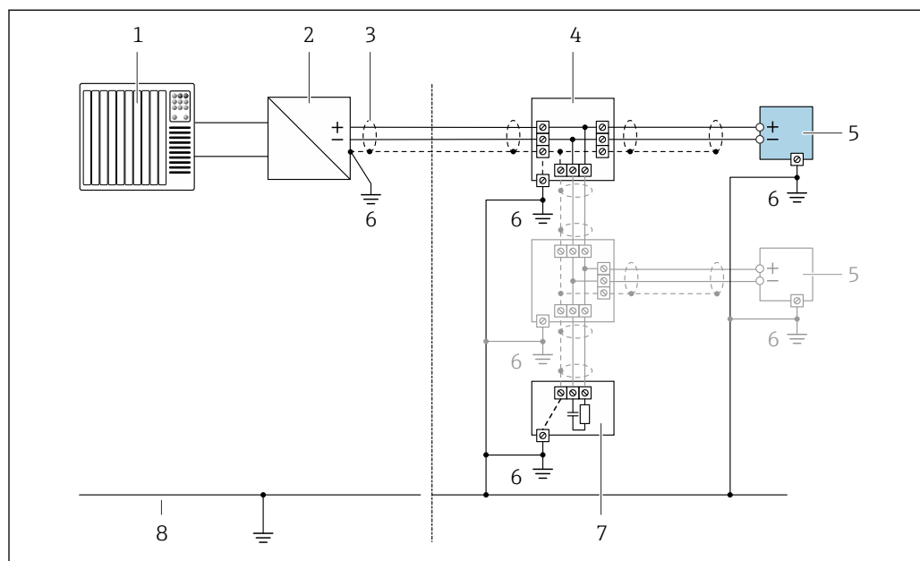
Fig. 15 Ejemplo de conexión para PROFIBUS PA
