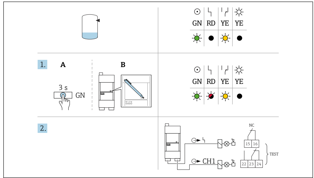
図 23 テスト/補正キー（緑色）を使用したエラーのシミュレーション
