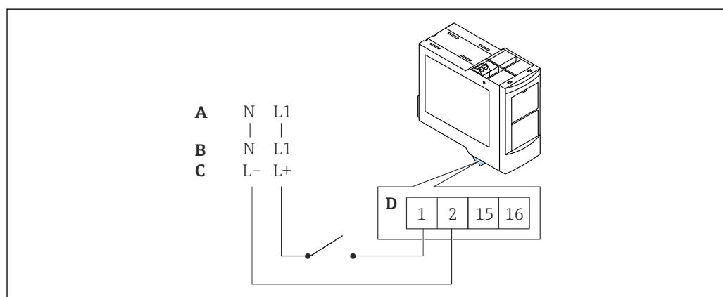
図 8 端子の配置
