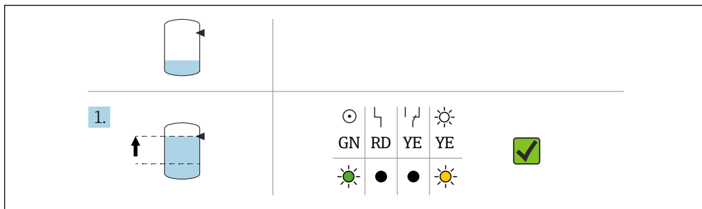
17 校正の確認
