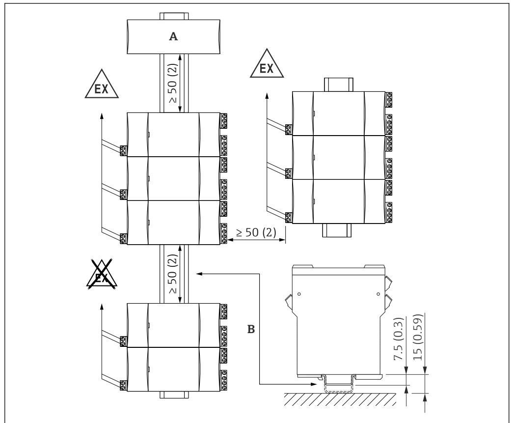
4 垂直取付の場合の最小距離
