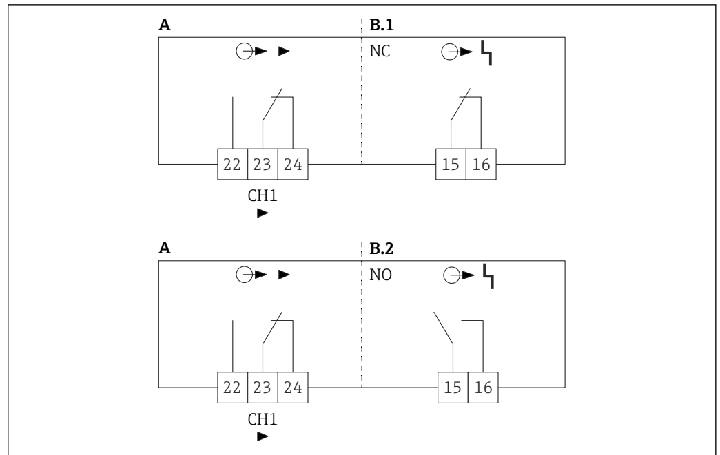
図 9 出力の接続
