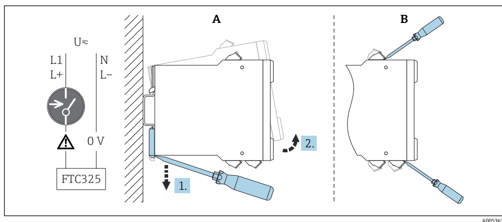
図 6 DIN レールからの取外し
