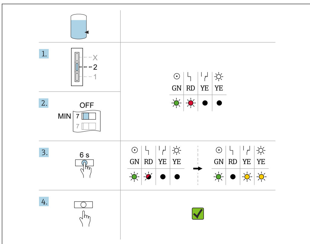
18 MIN（下限）アプリケーションの校正
