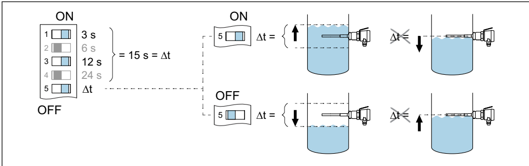
図 20 スイッチング遅延の設定例
