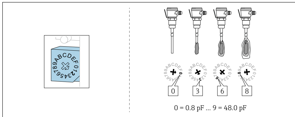
図 21 16 段階の感度設定
