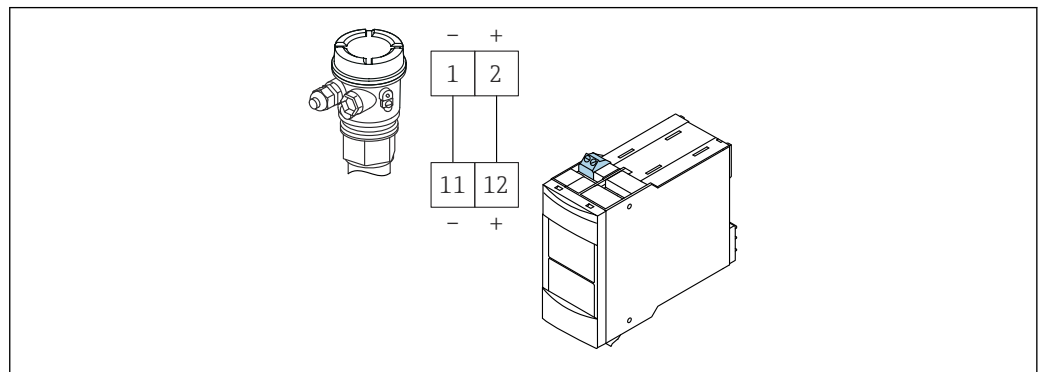
図 7 電源とセンサの接続
