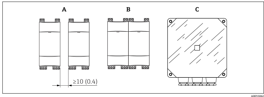
図 2 複数機器の設置。測定単位 mm (in)
