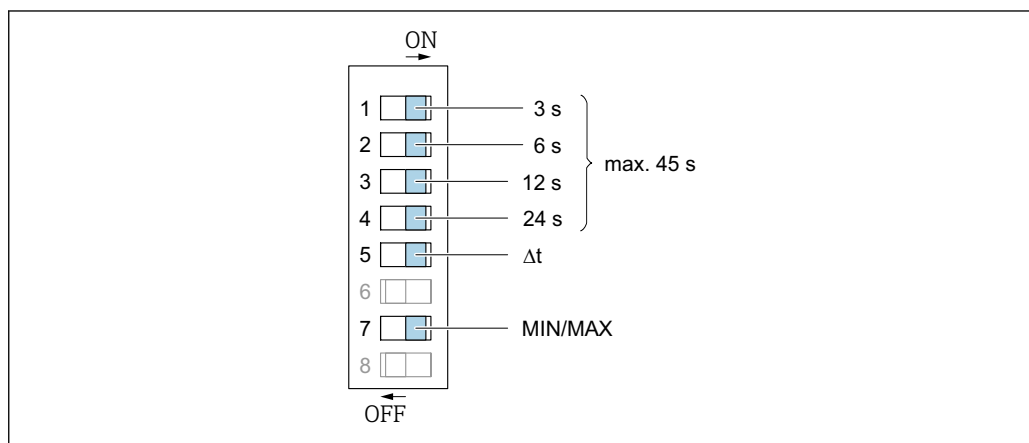
図 12 DIP スイッチ
