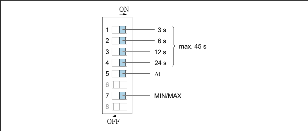
図 14 下限 (MIN) / 上限 (MAX) 設定用 DIP スイッチ
