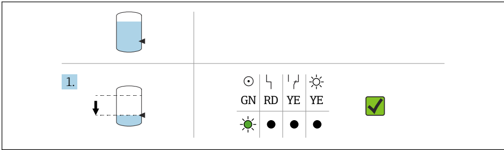
図 19 校正の確認
