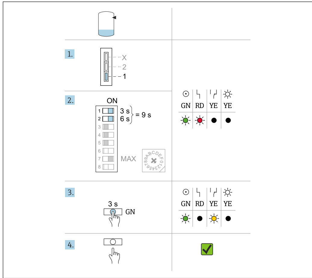
図 22 テスト/補正キー（緑色）を使用した変更の適用
