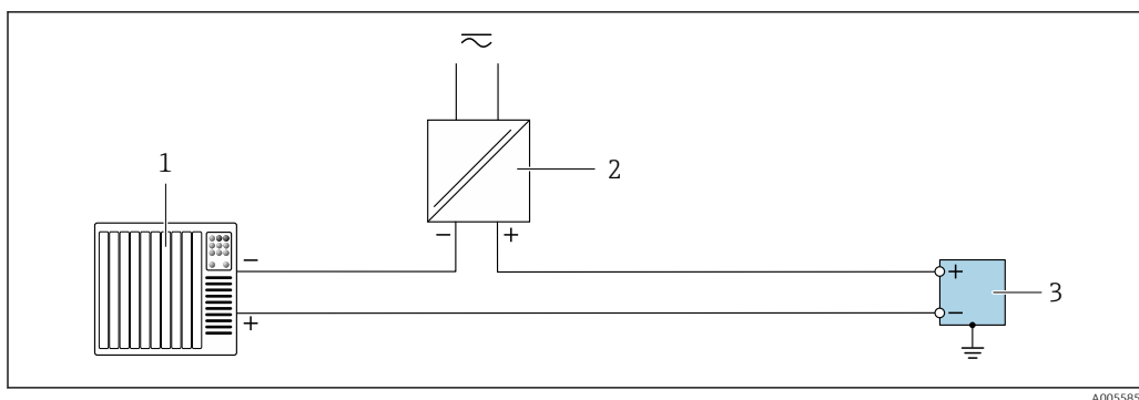
22 Пример подключения для импульсного/частотного/релейного выхода (пассивного)
