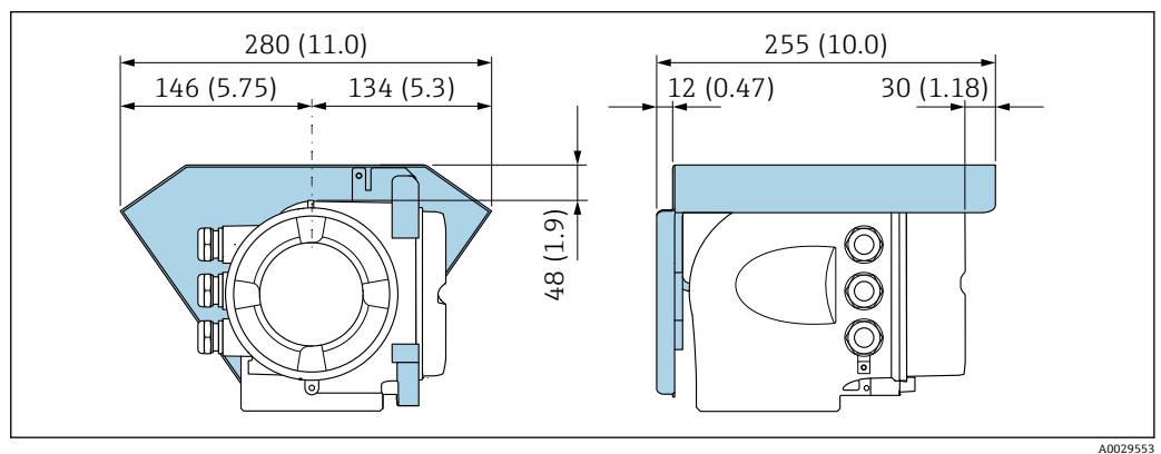
图 10 Proline 500 变送器的防护罩; 单位: mm (in)
