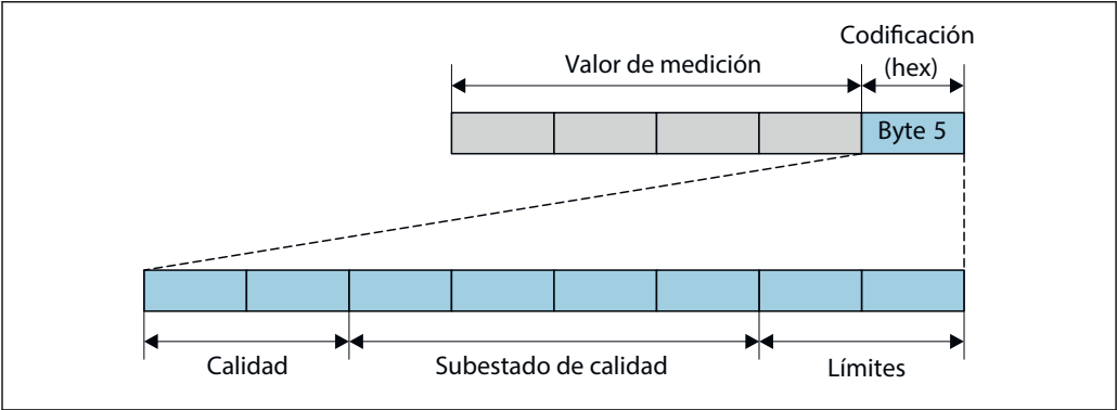
31 Estructura del byte de estado
