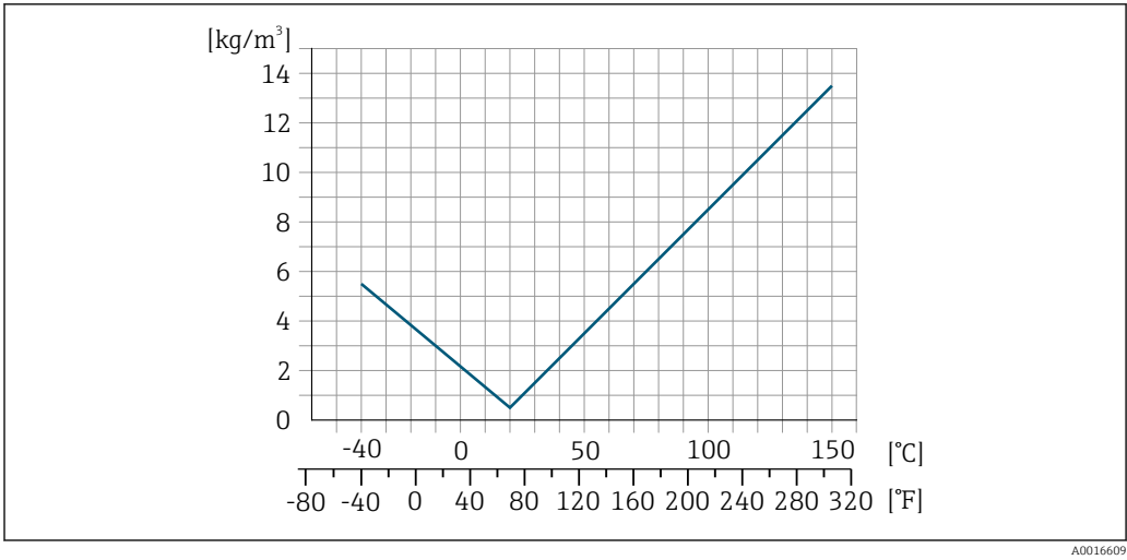
34 Ajuste en campo de la densidad, p. ej., a +20 °C (+68 °F)
