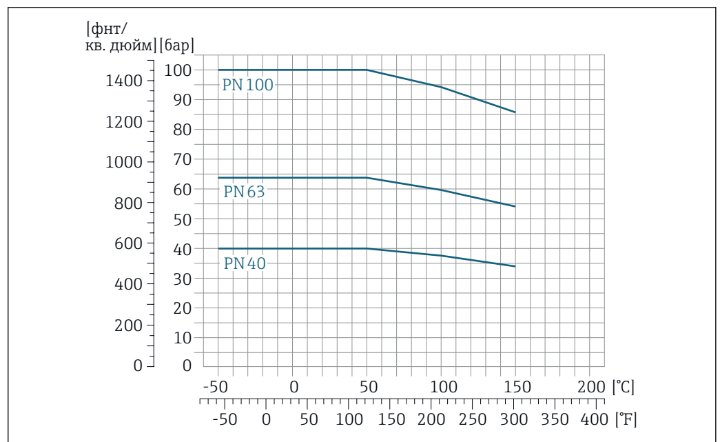
15 Материал фланца 1.4301 (304); смачиваемые компоненты: титан
