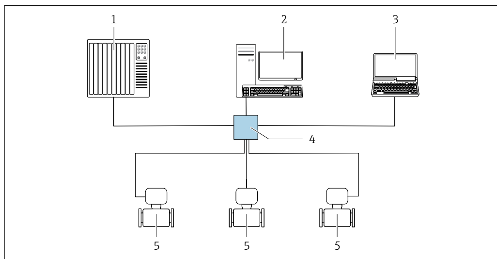
▣ 28 Варианты дистанционного управления через сеть EtherNet/IP: топология «звезда»
