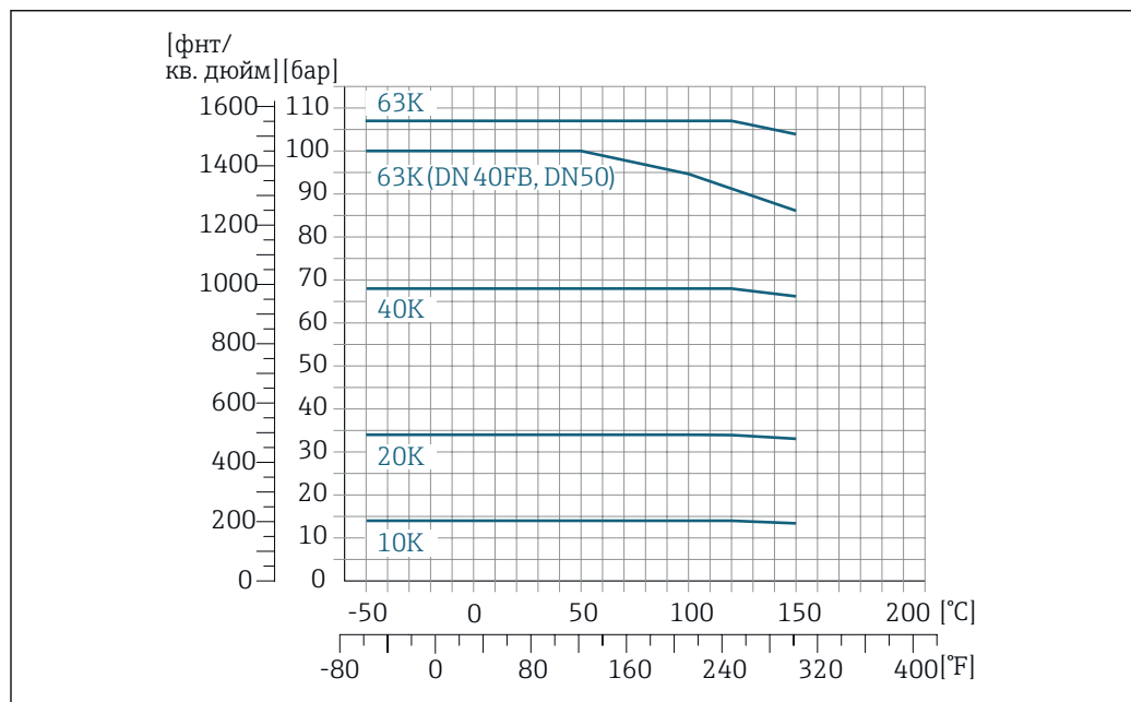
17 Материал фланца 1.4301 (304). Смачиваемые компоненты: титан.
