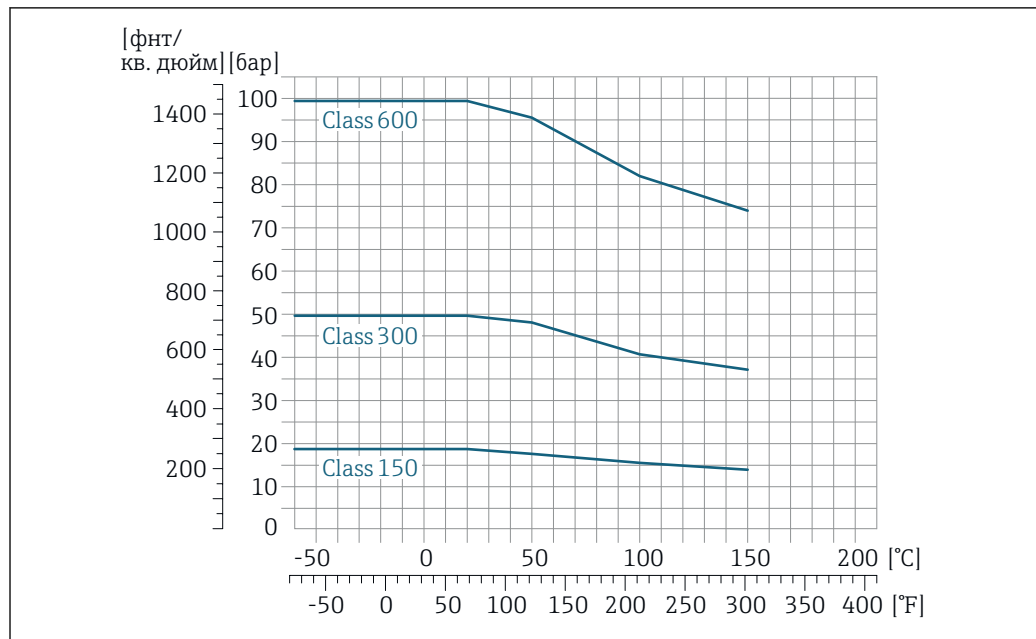
16 Материал фланца 1.4301 (304); смачиваемые компоненты: титан
