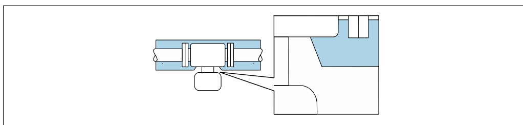
20 Aislamiento térmico con cuello de extensión expuesto
