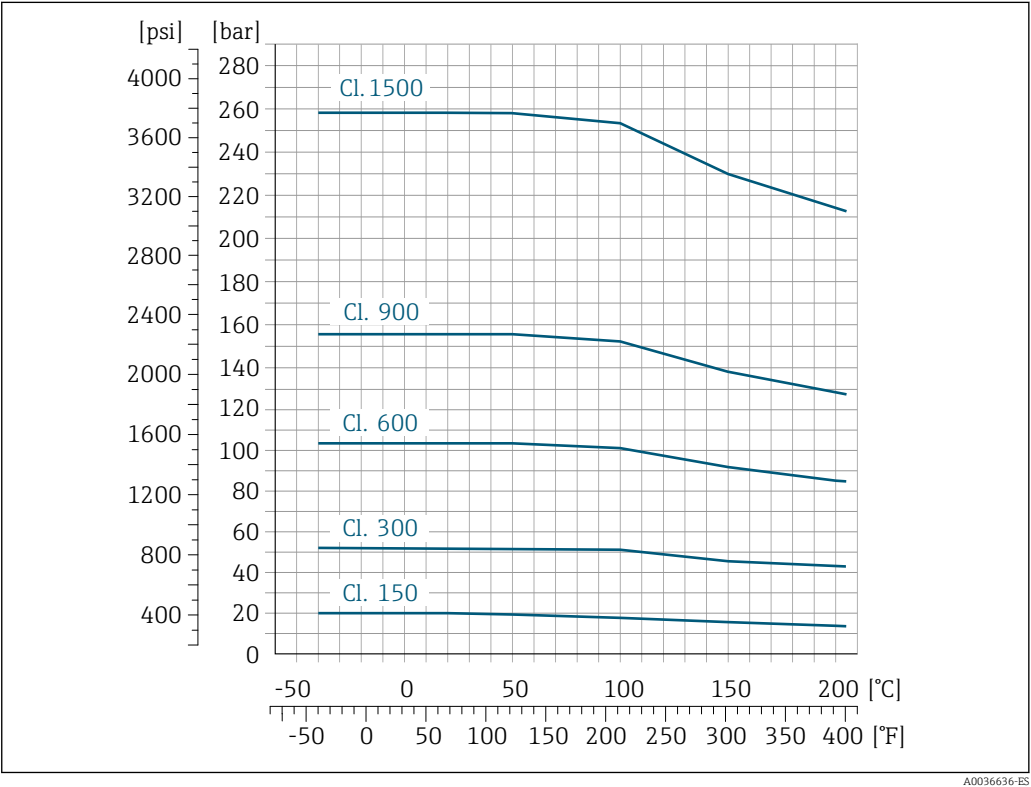
18 Con material de la brida acero inoxidable, 1.4410/F53 25Cr dúplex (superdúplex)
