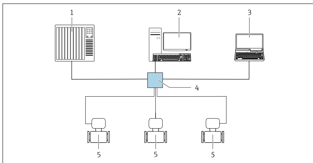
41 Opciones para la configuración a distancia mediante red EtherNet/IP: topología en estrella
