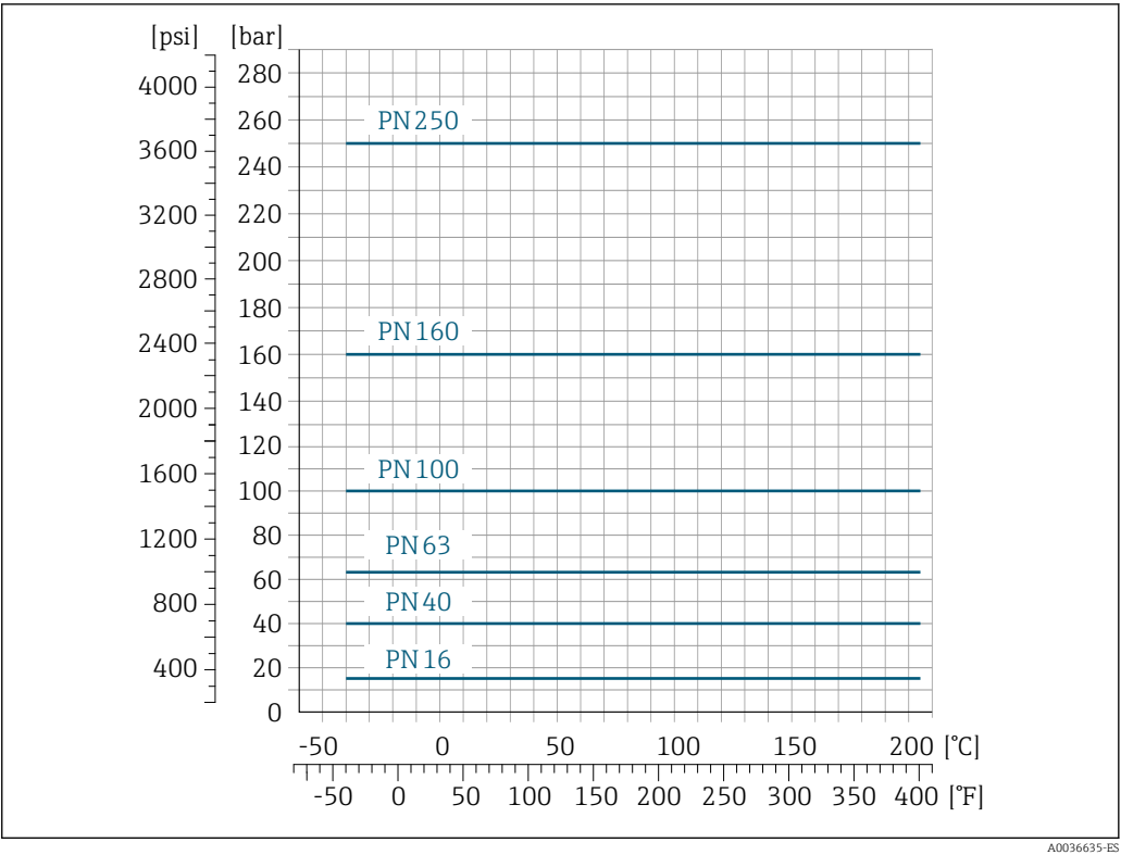
17 Con material de la brida acero inoxidable, 1.4410/F53 25Cr dúplex (superdúplex)
