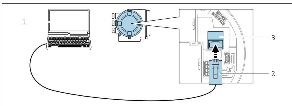
45 Conexión mediante la interfaz de servicio (CDI-RJ45)
